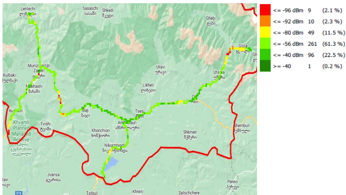
RX_LEV, სილქნეტი
