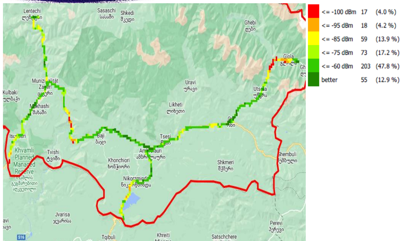
RSCP, სილქნეტი
