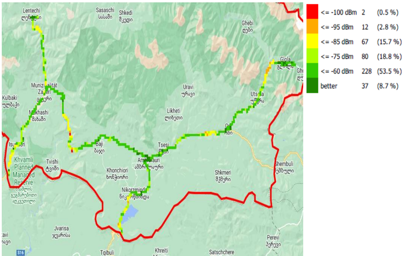
RSCP, მაგთიკომი
