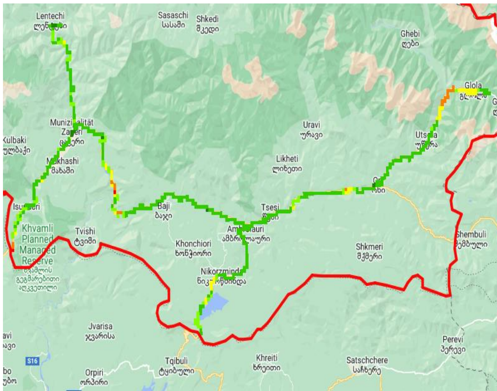
RSRP, სილქნეტი
