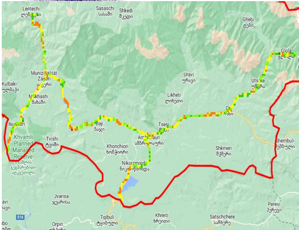
RSRQ, მაგთიკომი
