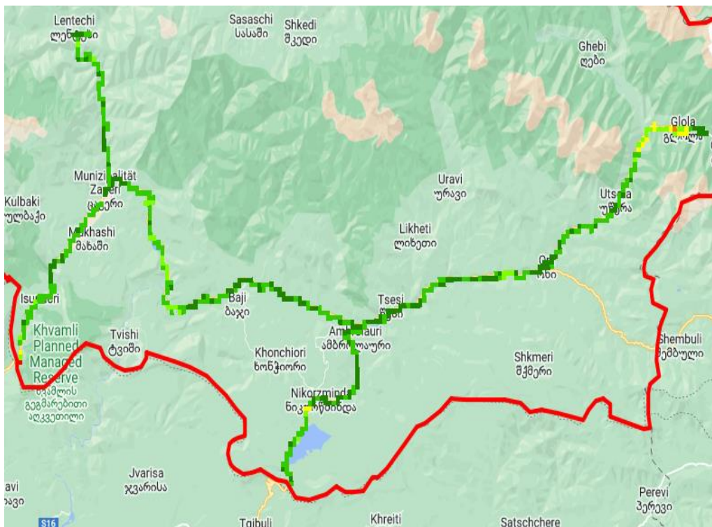
C/I, სილქნეტი
