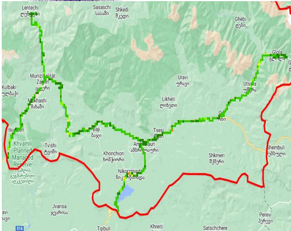
C/I, მაგთიკომი
