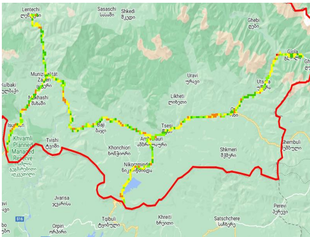
RSRQ, სილქნეტი
