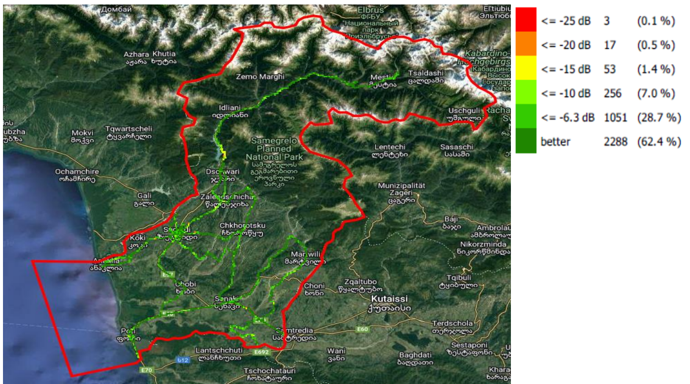
Ec/Io, სილქნეტი
