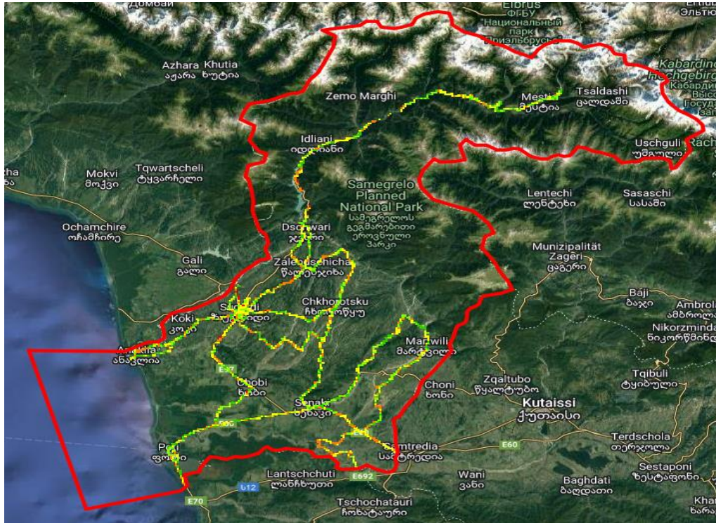
RSRQ, სილქნეტი
