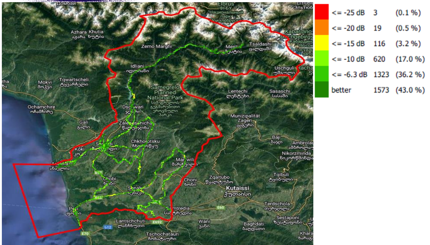
Ec/Io, მაგთიკომი
