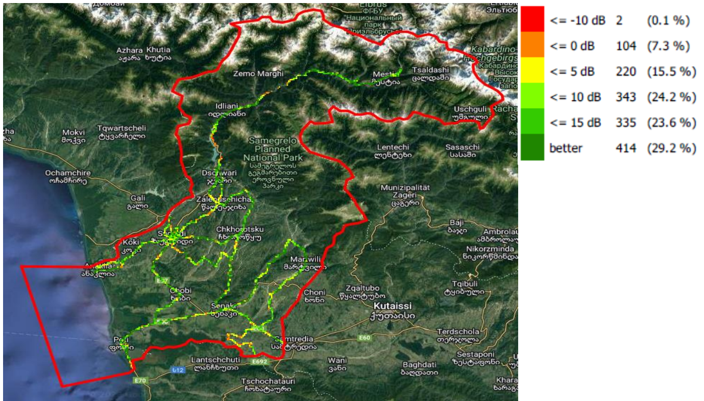
SINR, სილქნეტი
