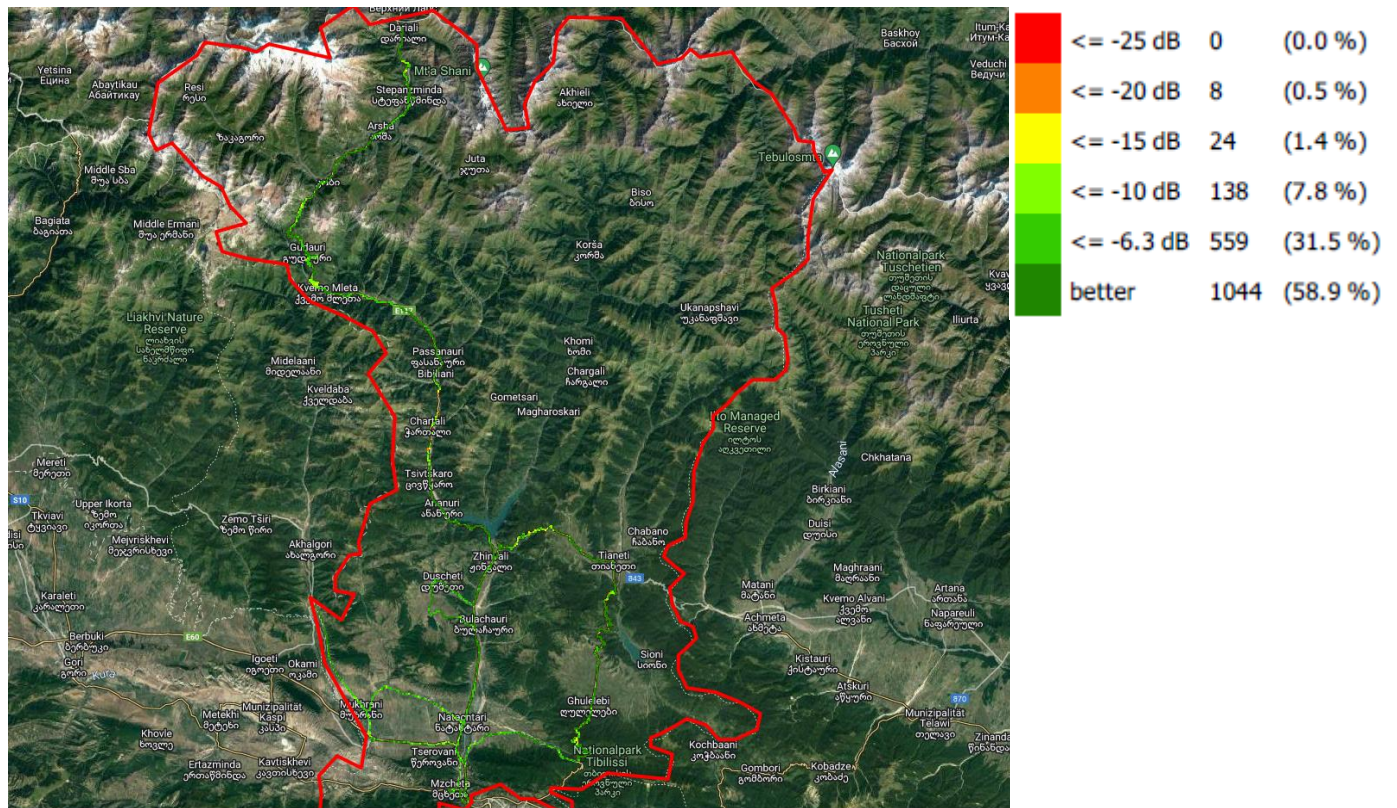
Ec/Io, ვიონი საქართველო
