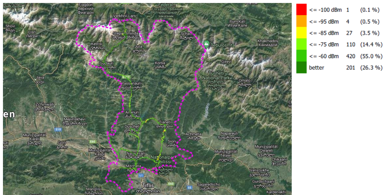
RSCP, მაგთიკომი
