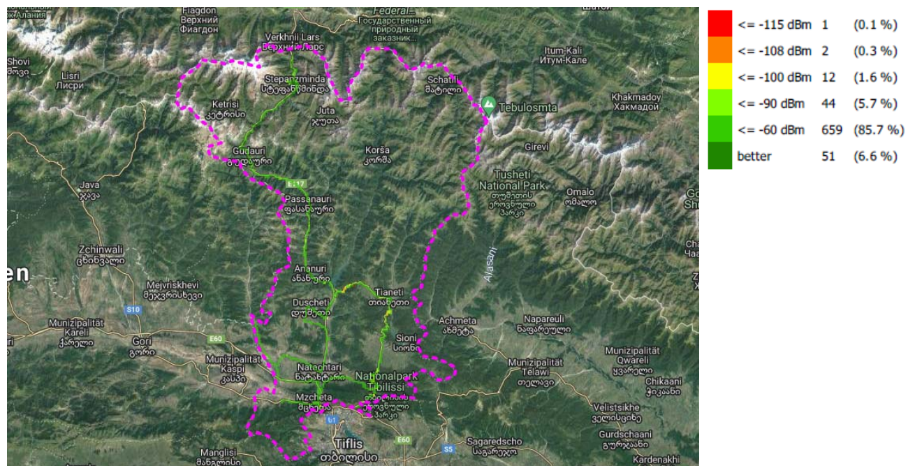
RSRP, მაგთიკომი
