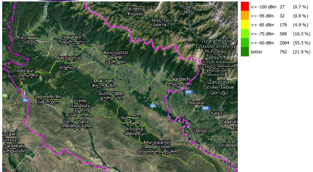
RSCP, მაგთიკომი
