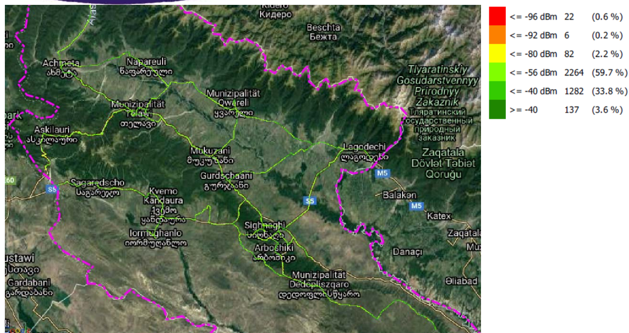
RX_LEV, სილენეტი
