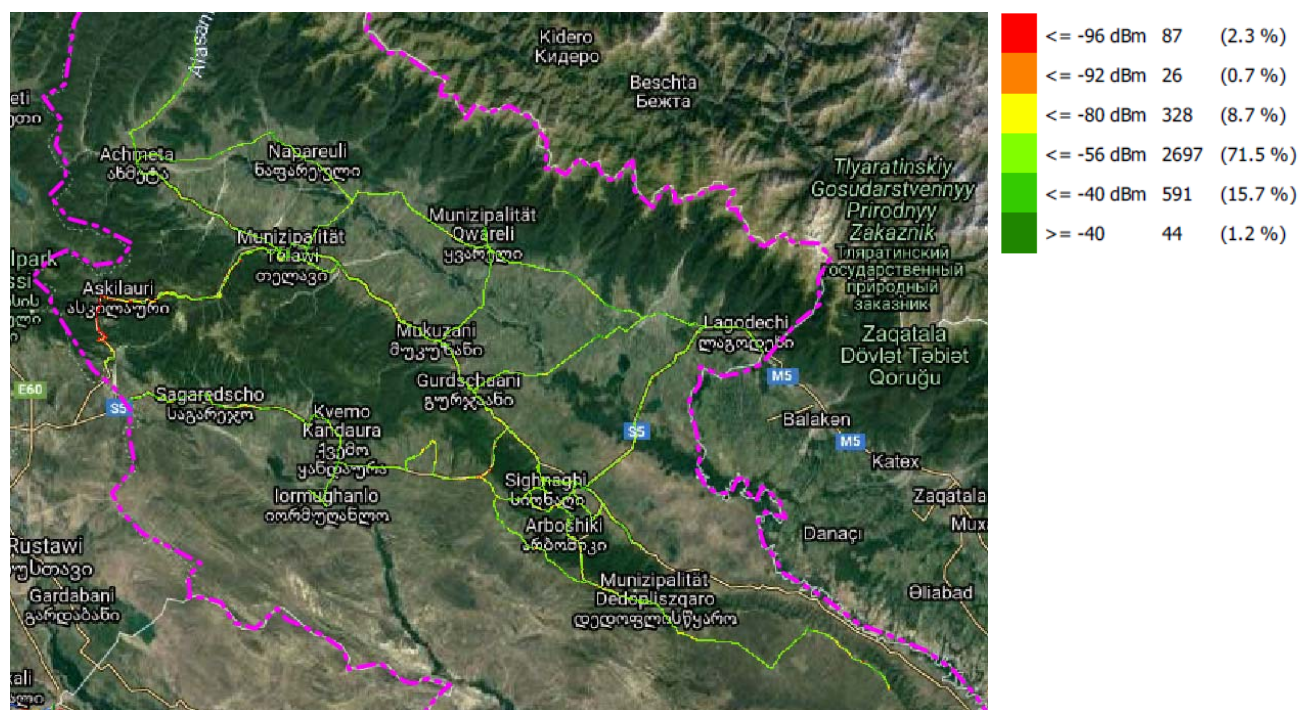
RX_LEV, ვიონი საქართველო
