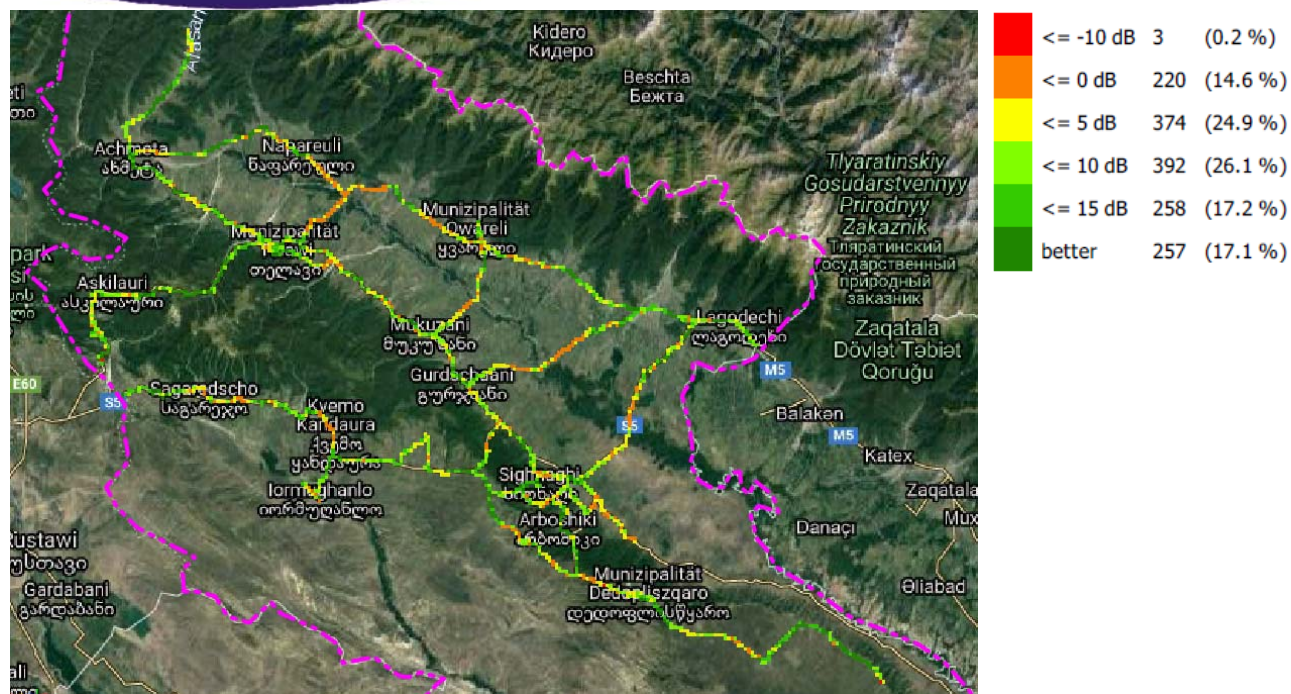
SINR, სილქნეტი
