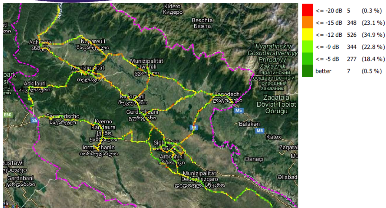
RSRQ, მავთიკომი
