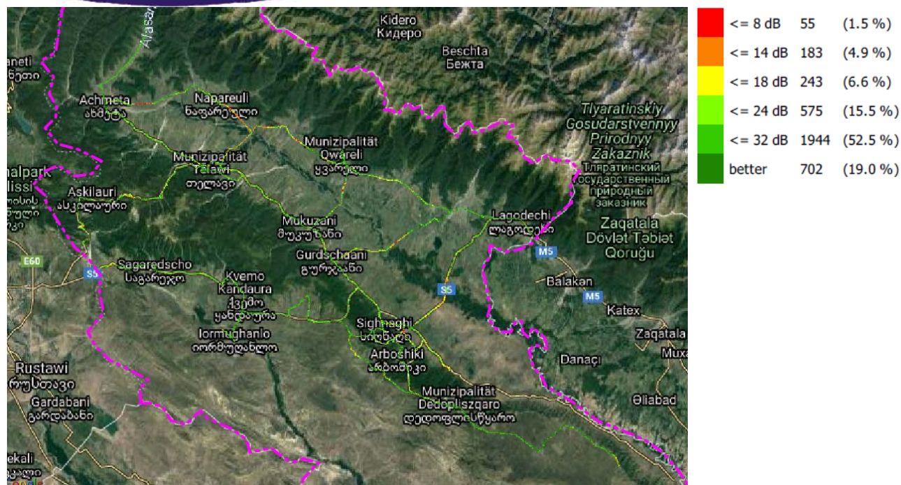
C/I, მაგთიკომი
