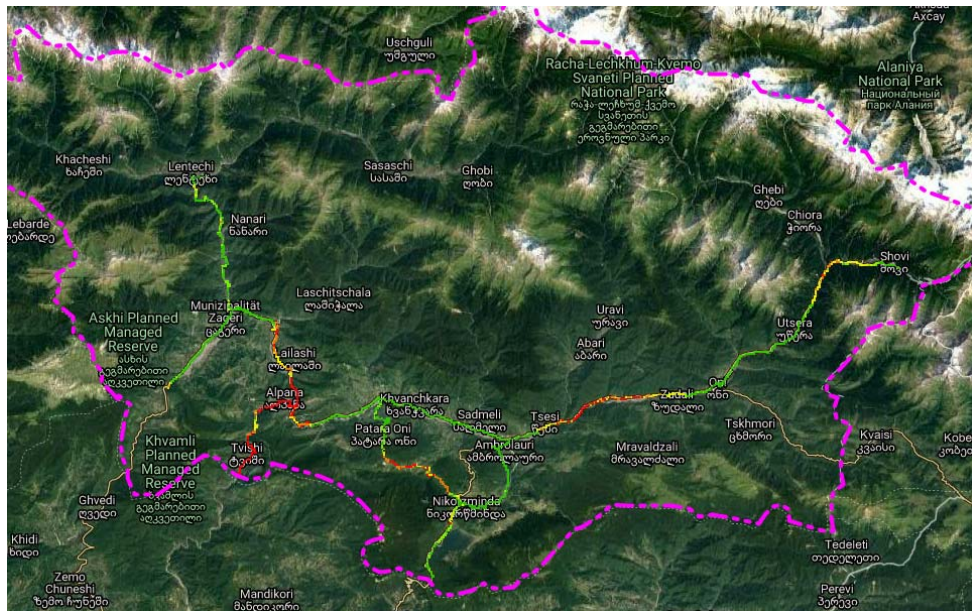
RSRP, სილქნეტი
