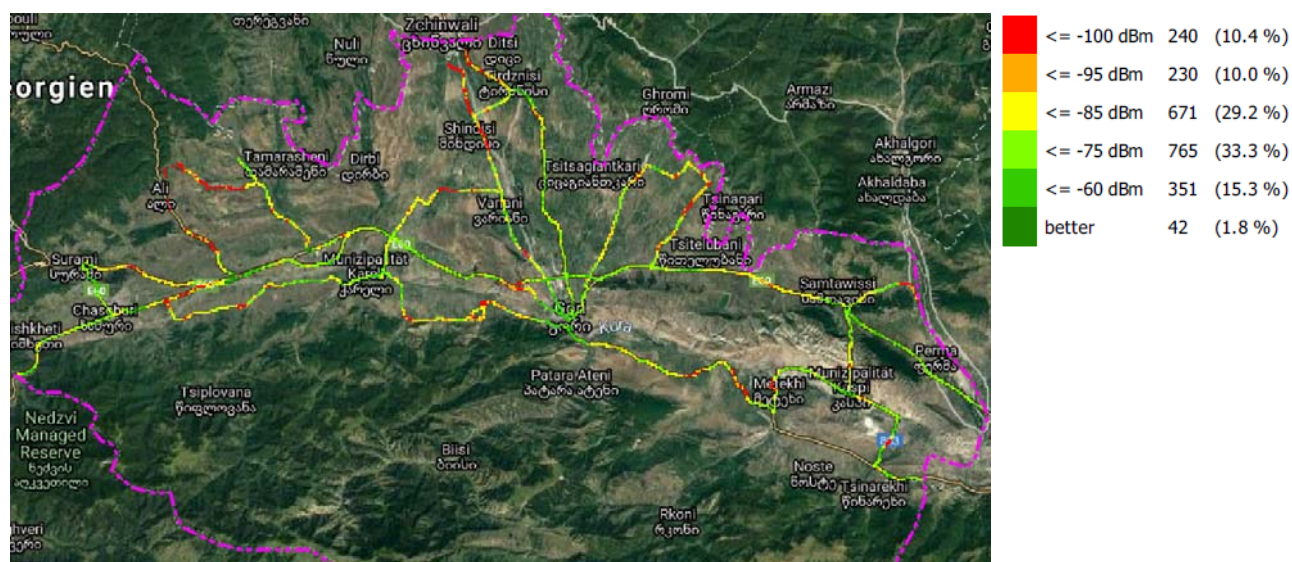
RSCP, ვიონი საქართველო
