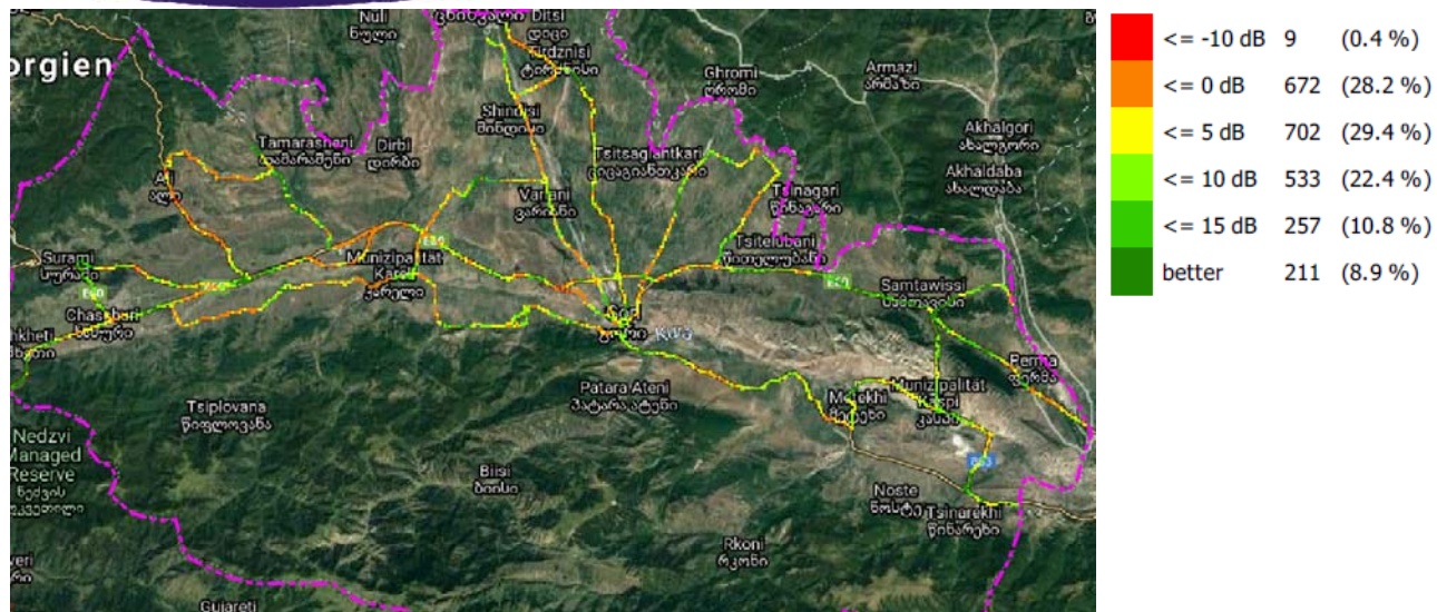
SINR, ვიონი საქართველო
