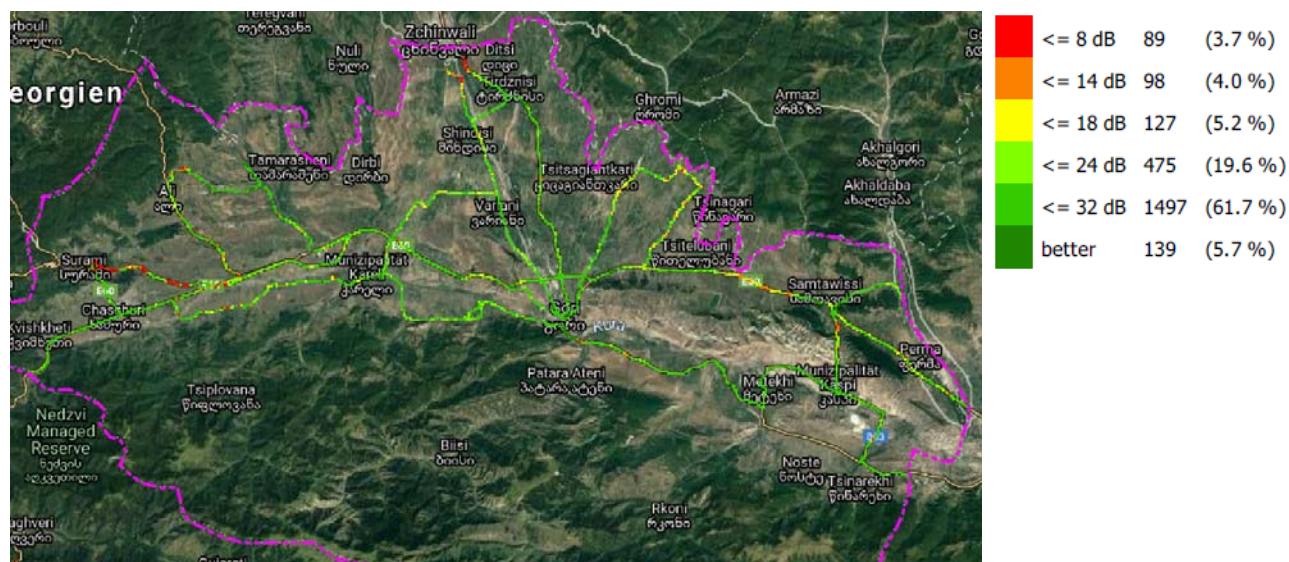
C/I, ვიონი საქართველო
