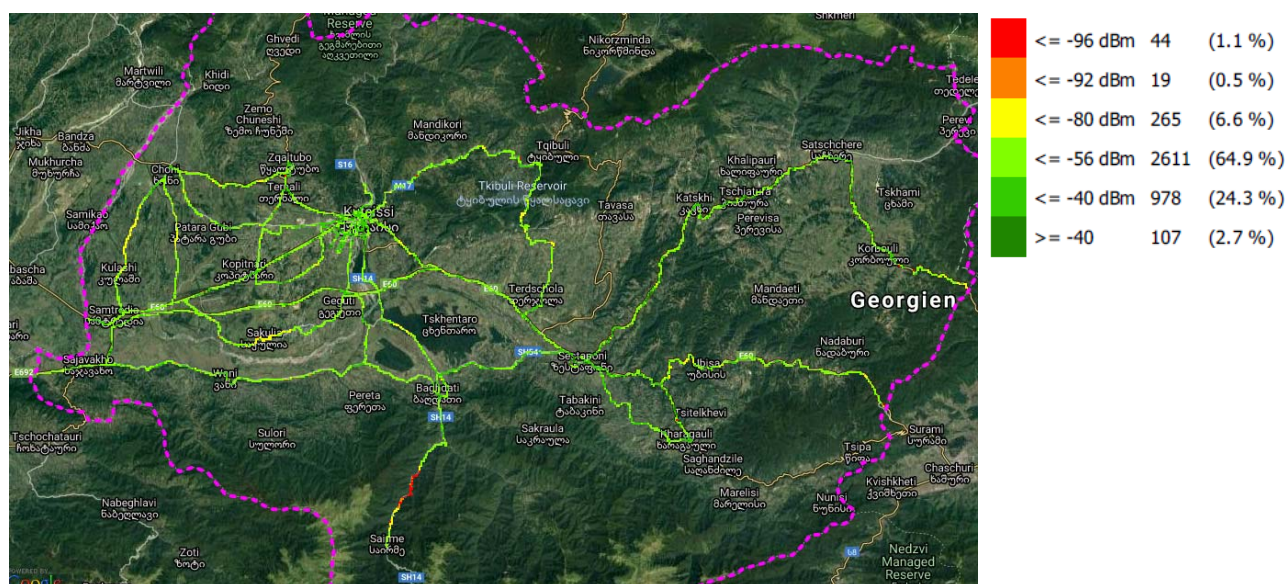
RX_LEV, სილქნეტი
