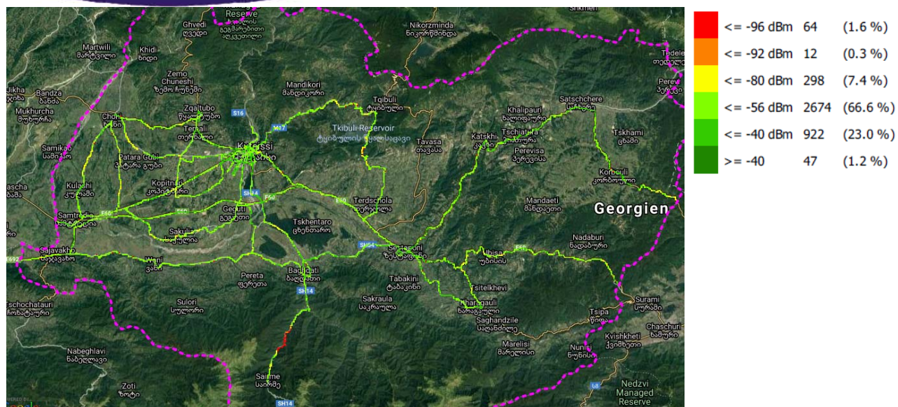
RX_LEV, მატეოკომი
