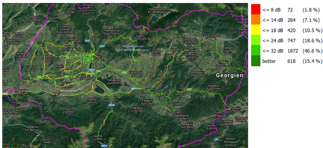
C/I, მაგთიკომი
