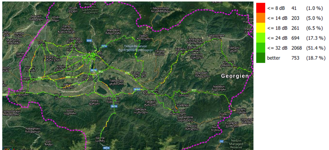
C/I, სილქნეტი
