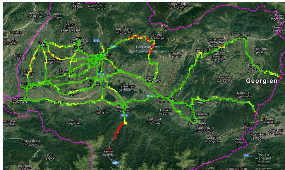
RSRP, სილქნეტი
