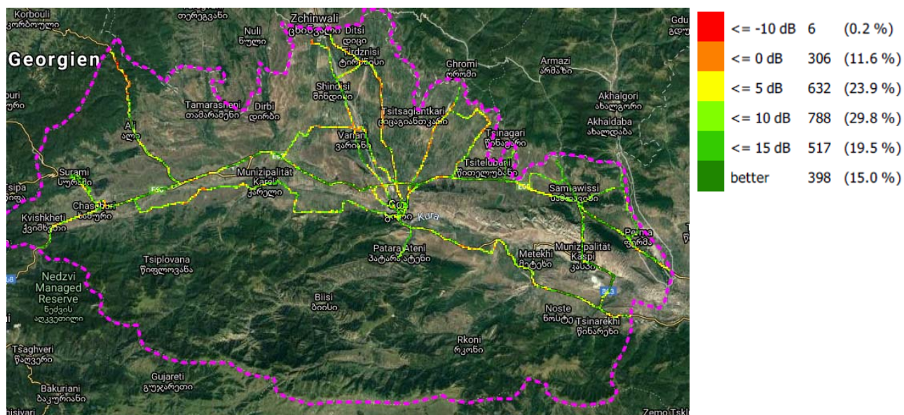
SINR, სილქნეტი
