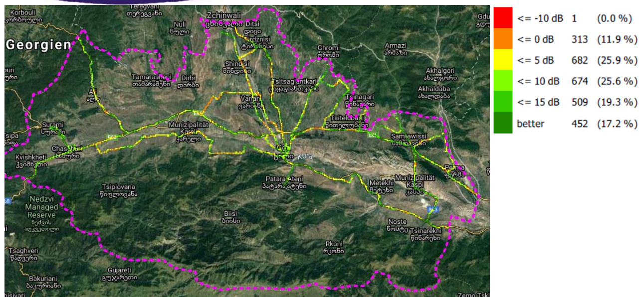
SINR, მაგთიკომი
