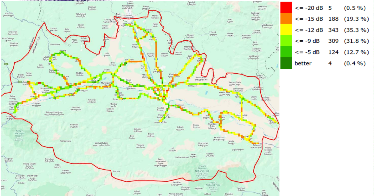
RSRQ, სოლქნეტი
