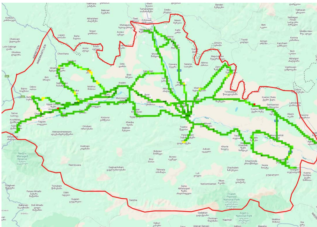
RSRP, სილქნეტი
