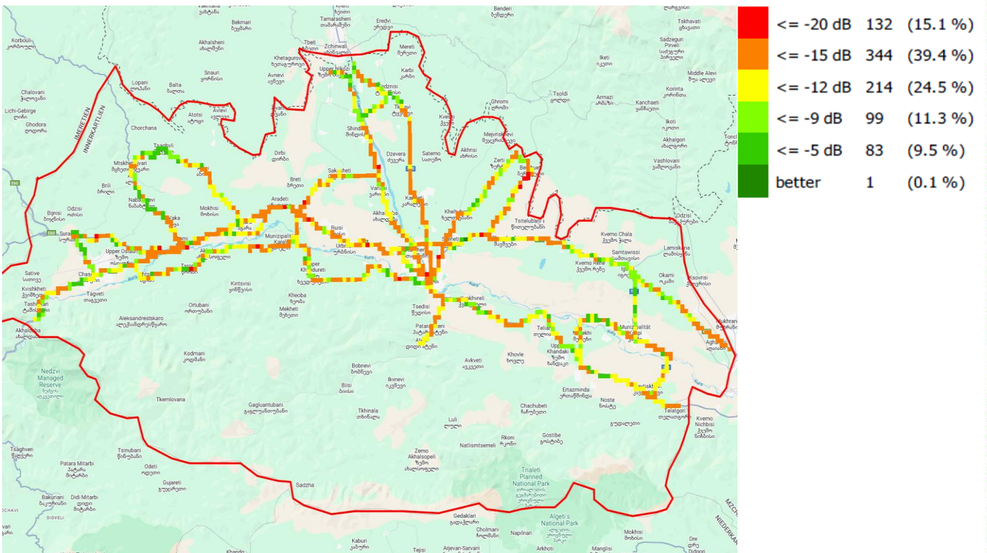
RSRQ, სელფი
