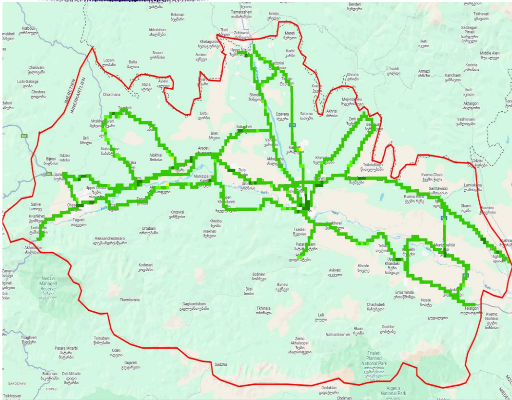
RSRP, მაგთიკომი
