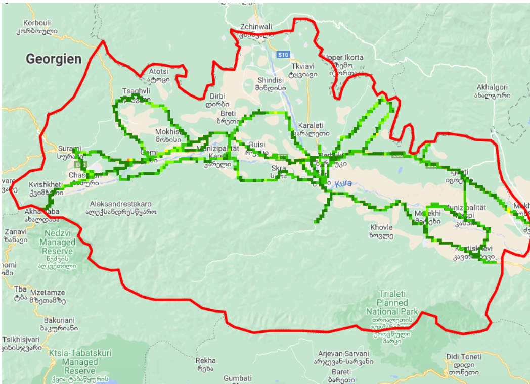
Ec/Io, სილქნეტი
