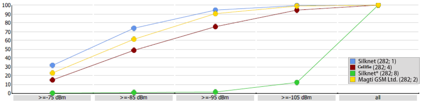
RSRP, სელვი
