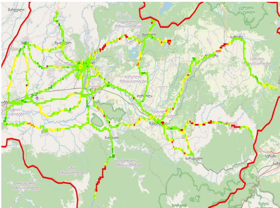
RX_LEV, სელფი
