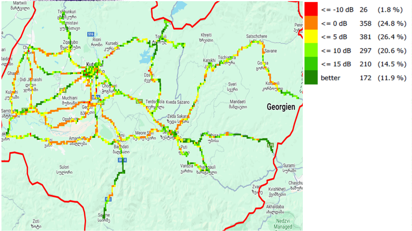
SINR, სელფი
