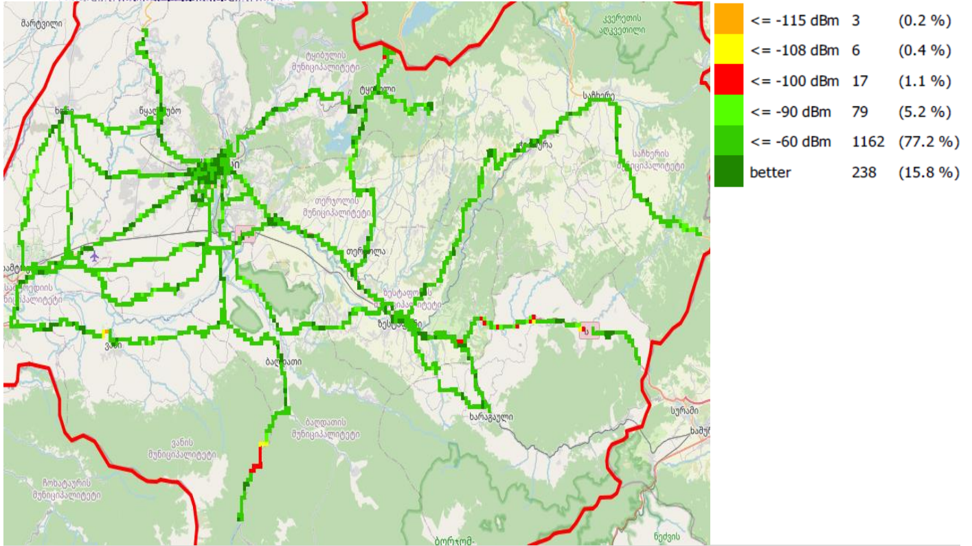
RSCP, სილქნეტი
