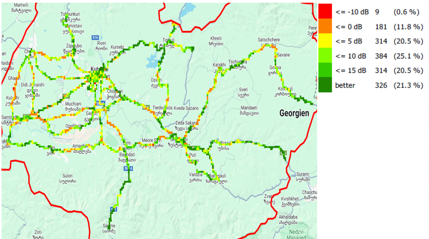
SINR, სილქნეტი
