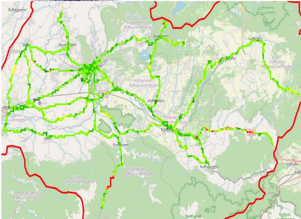
RX_LEV, სილქნეტი
