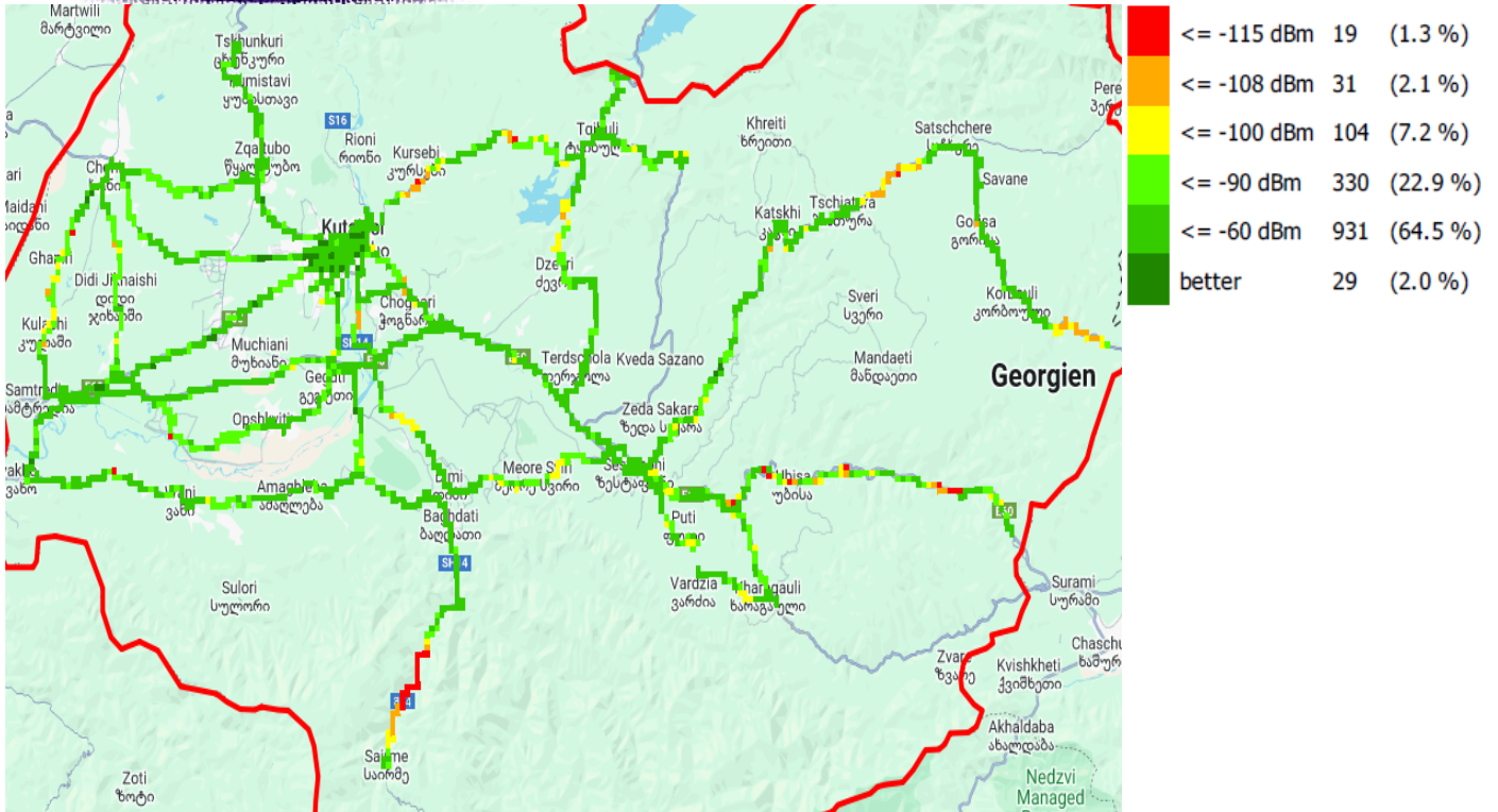
RSRP, სელფი
