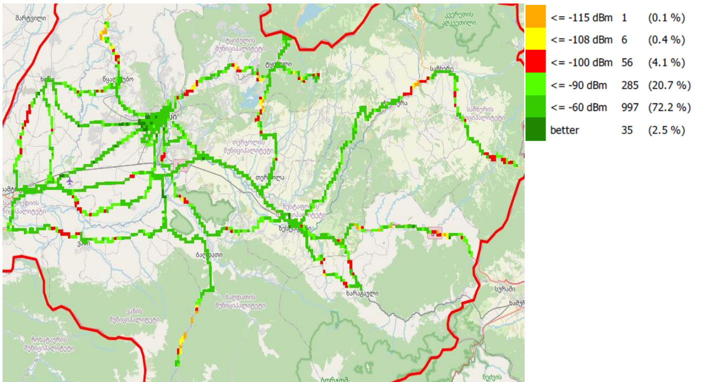
RSCP, სელვი
