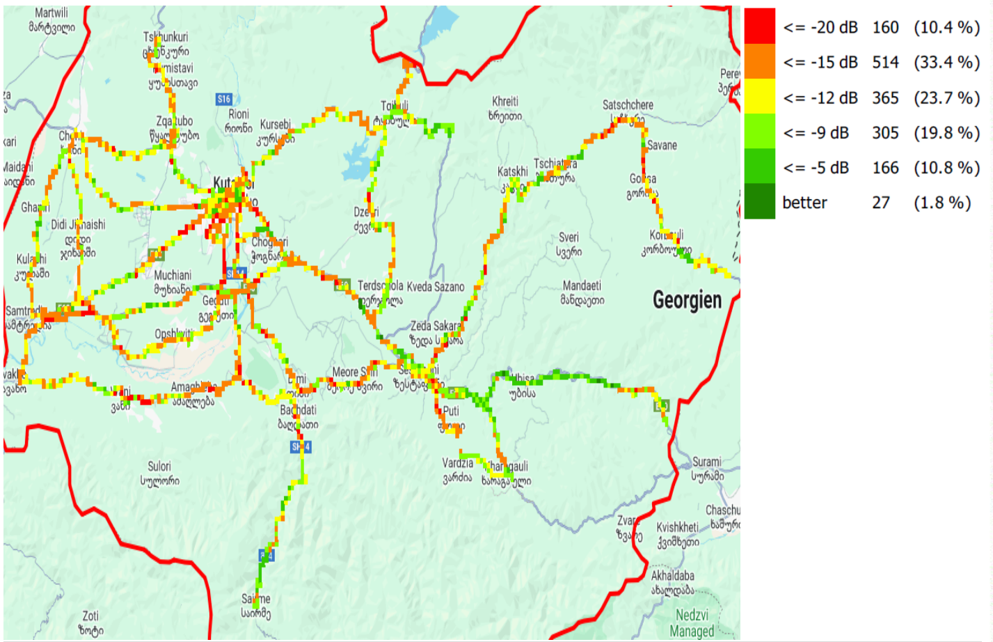
RSRQ, მაგთიკომი
