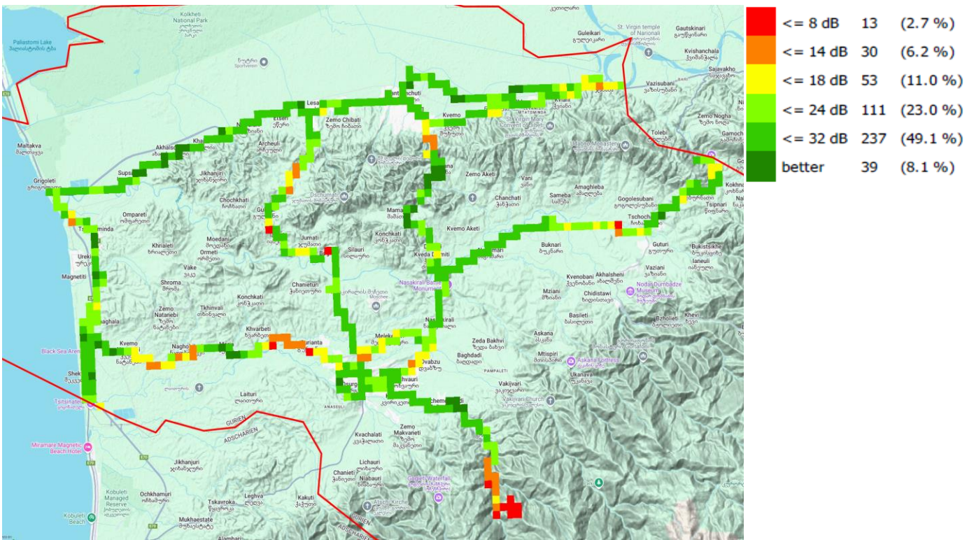
C/I, სილქნეტი
