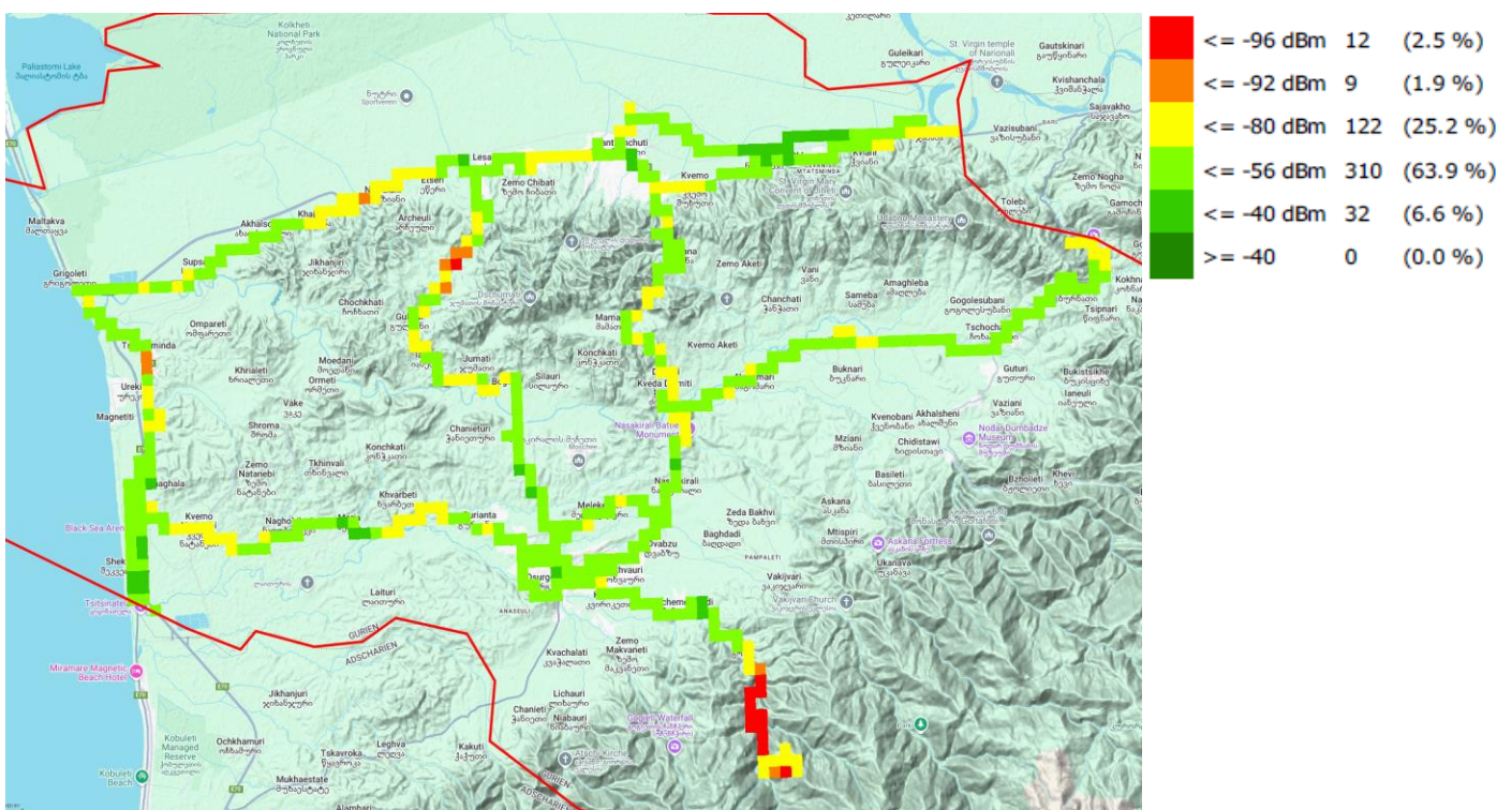
RX_LEV, სელი
