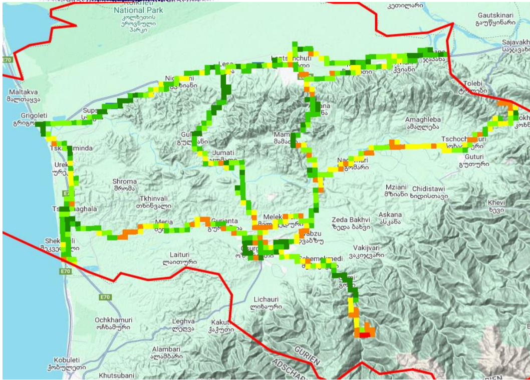
SINR, მაგთიკომი
