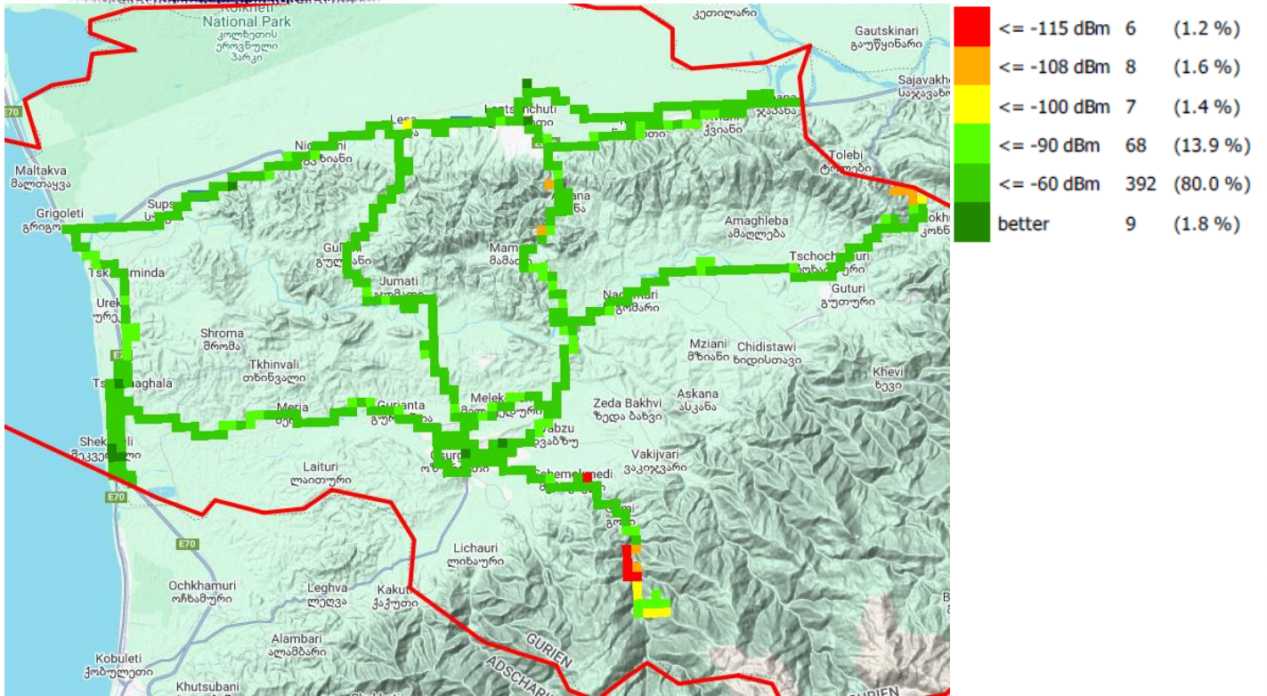
RSRP, მაგთიკომი
