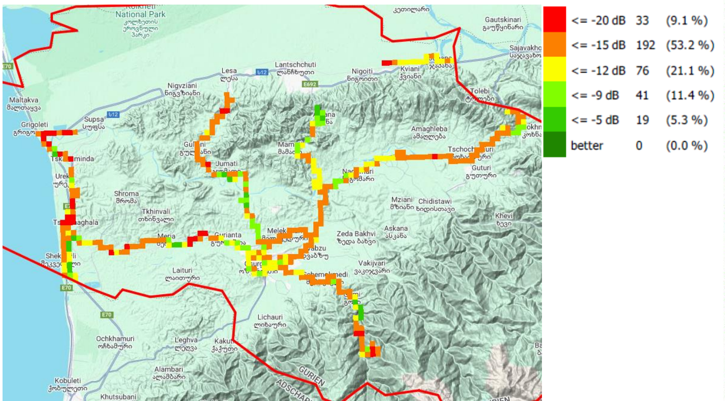
RSRQ, სელგი
