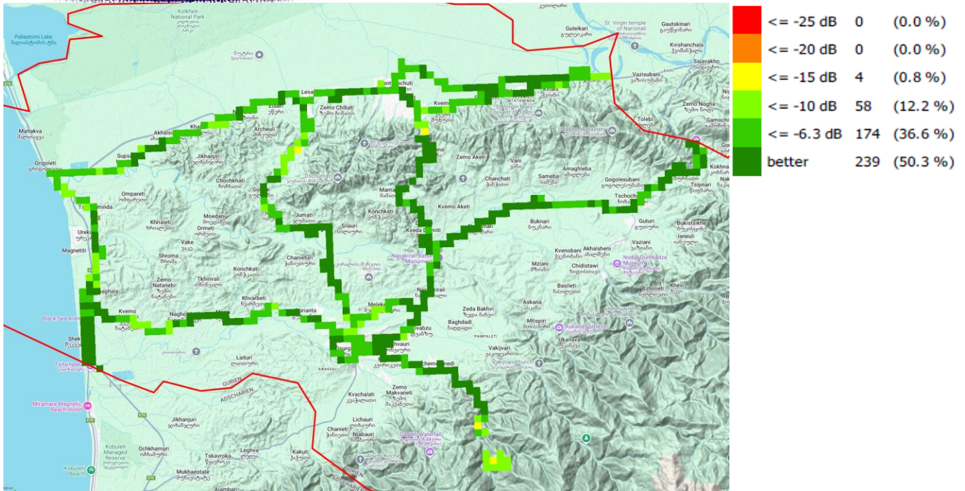
Ec/Io, სელები
