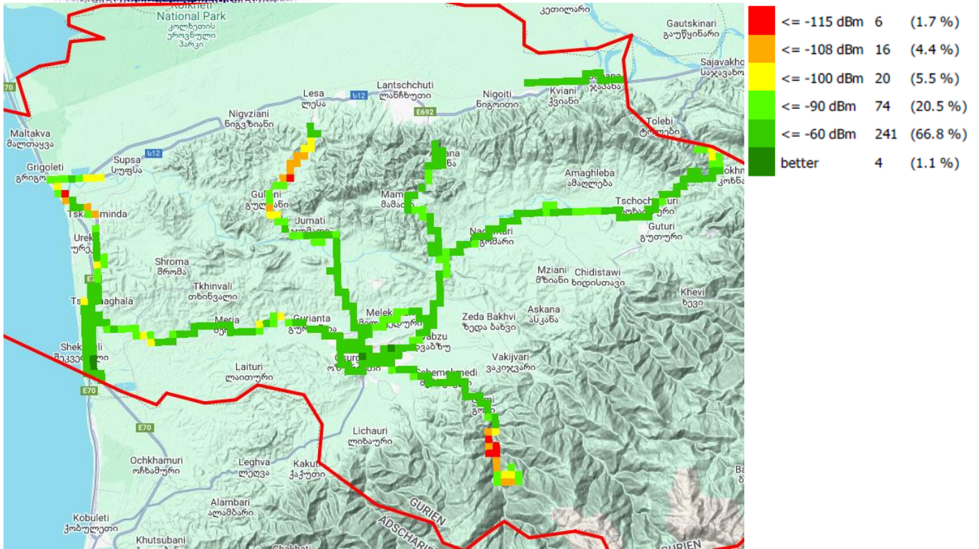
RSRP, სელფი
