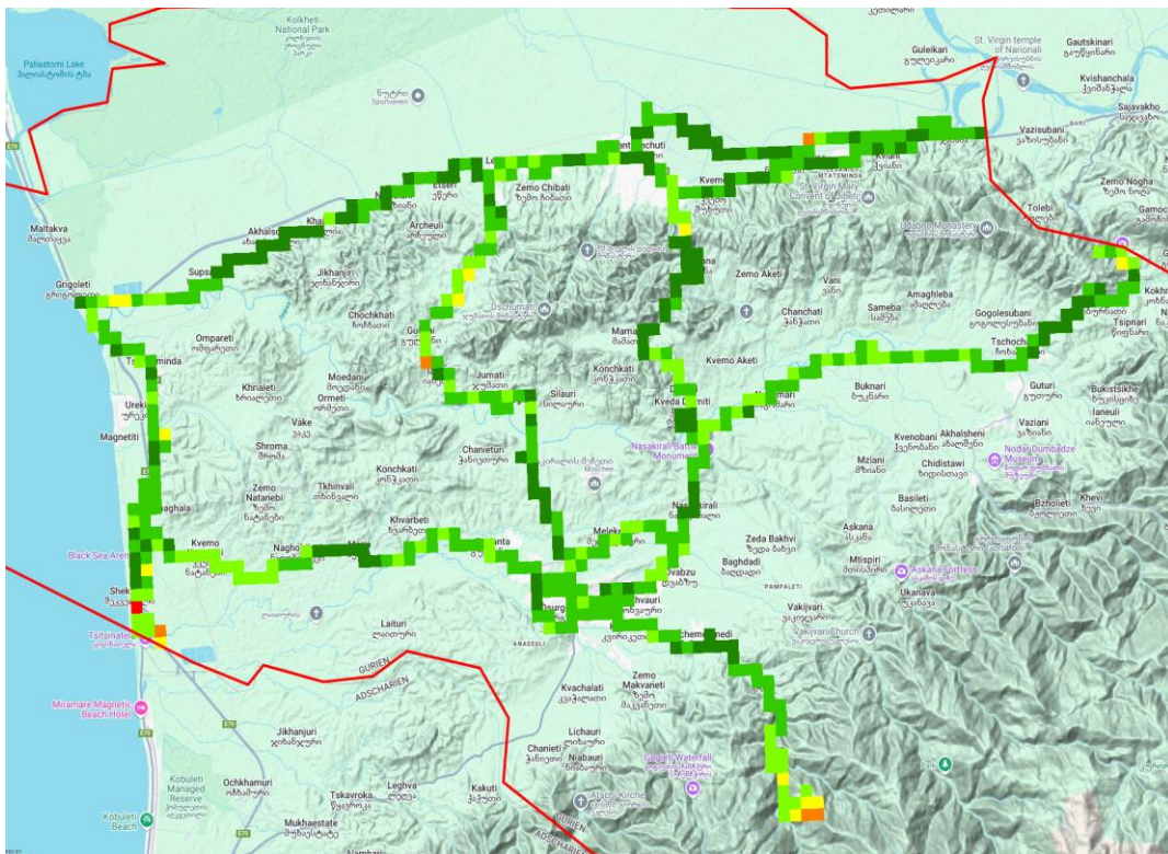
Ec/Io, სოლენეტი
