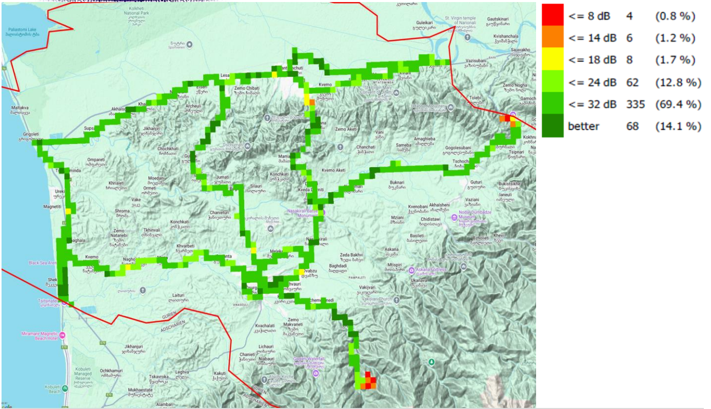
C/I, მგეტიკომი
