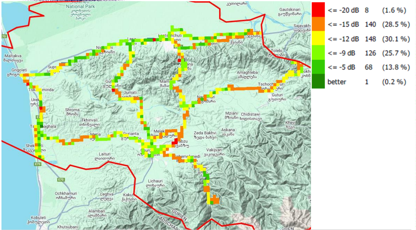
RSRQ, სილქნეტი
