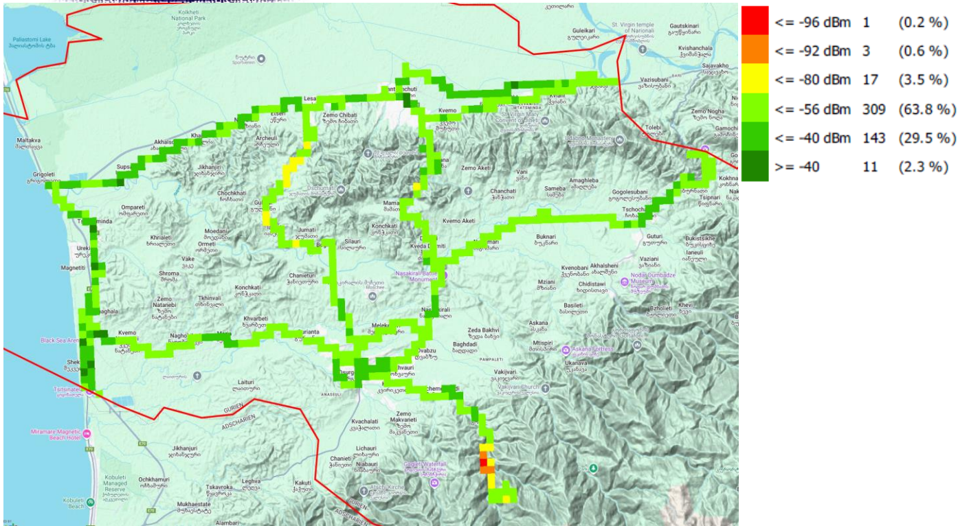
RX_LEV, სოლენგეტი
