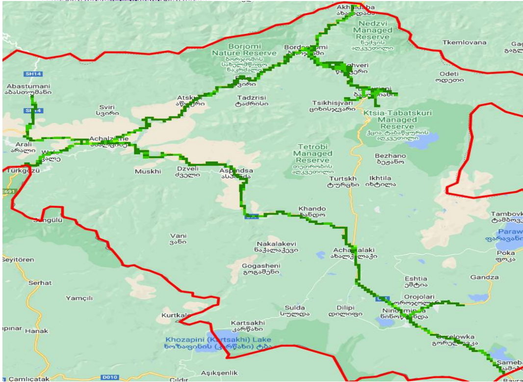
Ec/Io, მაგთიკომი
