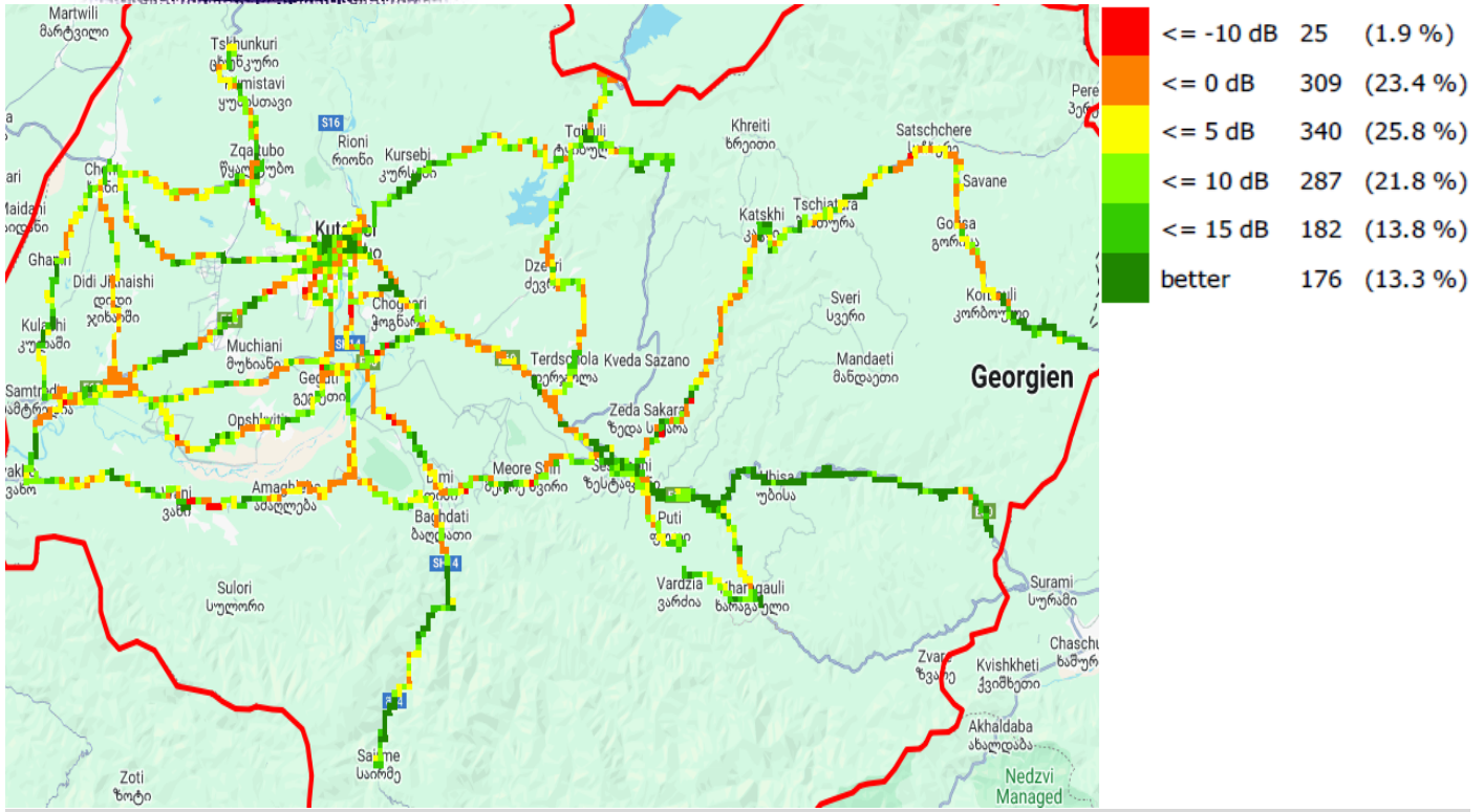
SINR, მათეკომი
