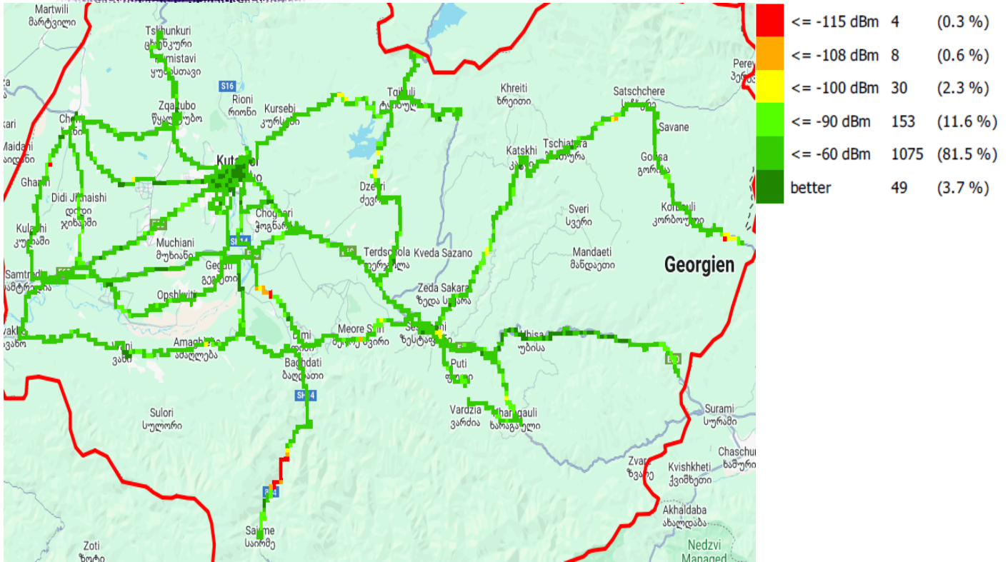
RSRP, მათეკომი
