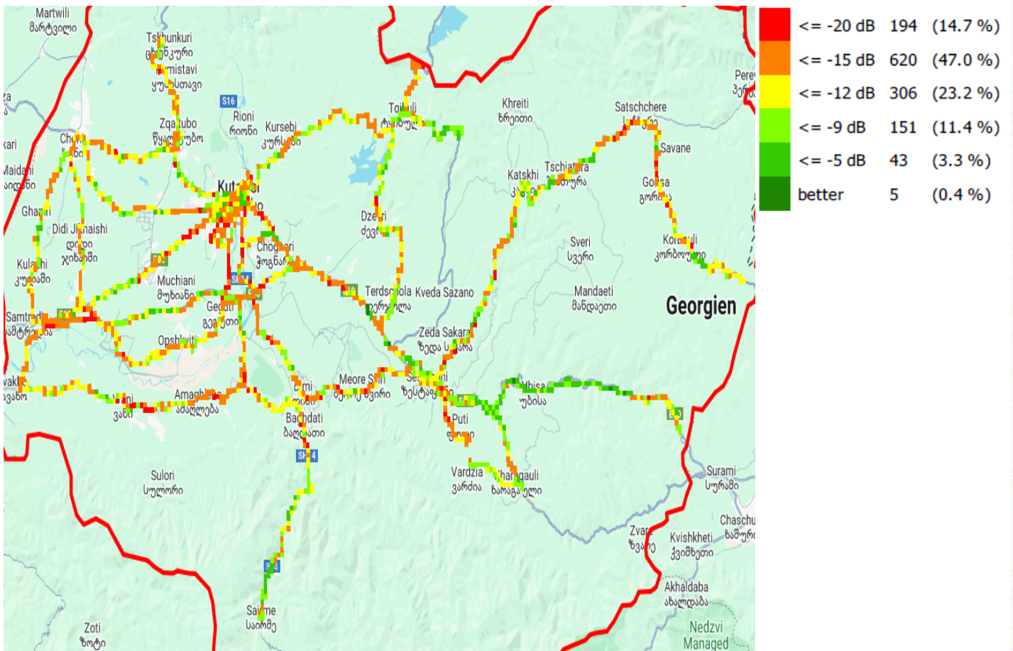
RSRQ, მაგთიკომი
