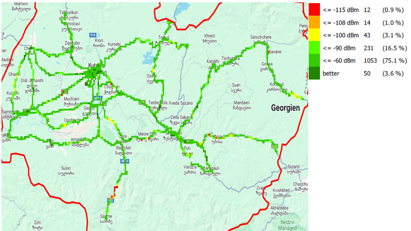
RSRP, სილქნეტი
