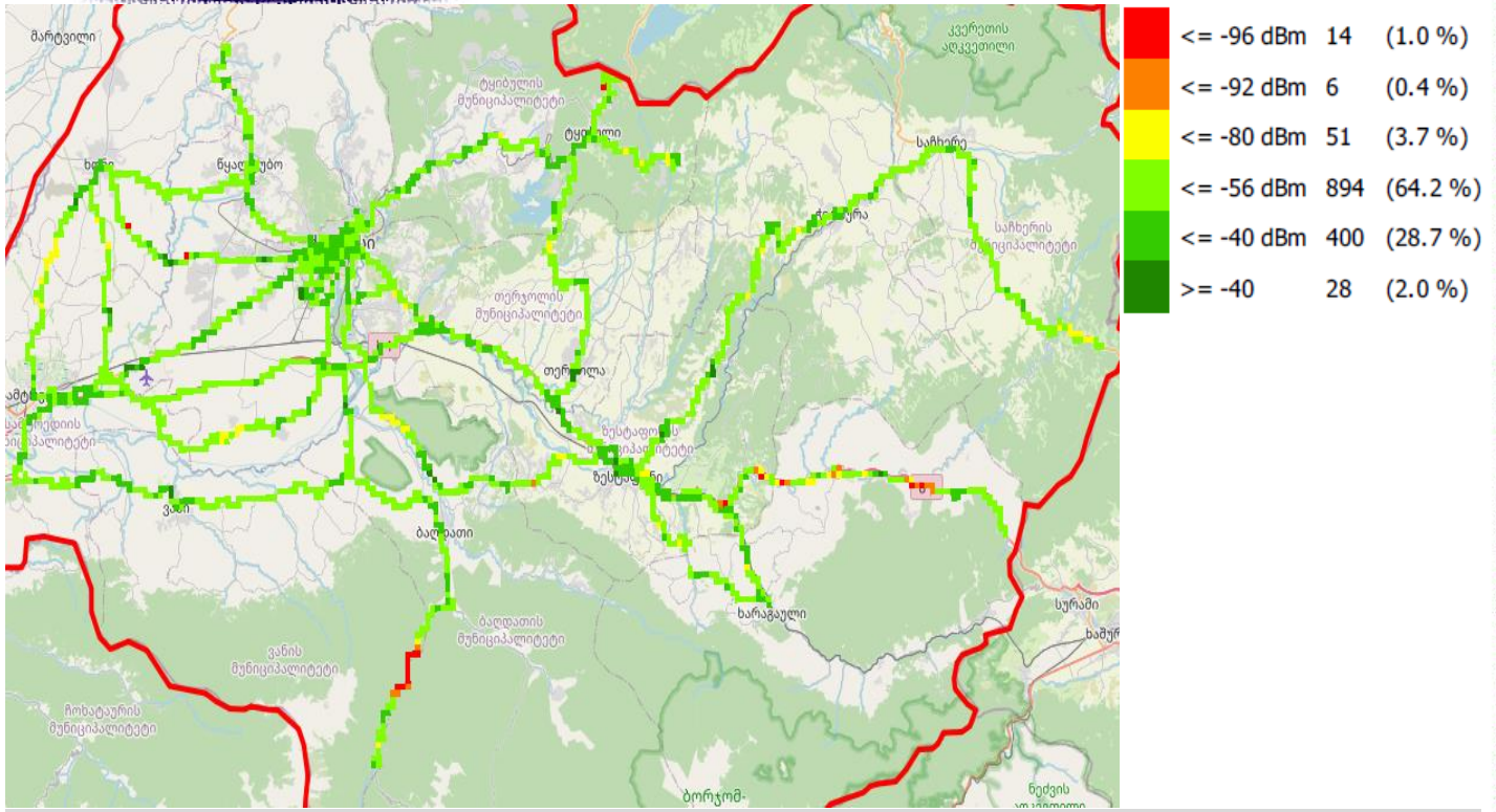
RX_LEV, სილქნეტი
