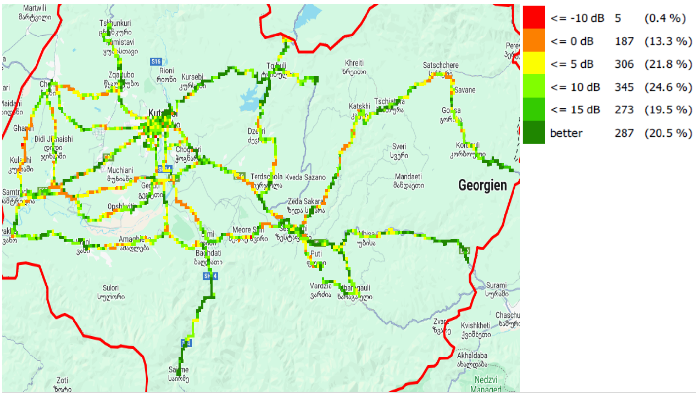
SINR, სილქნეტი
