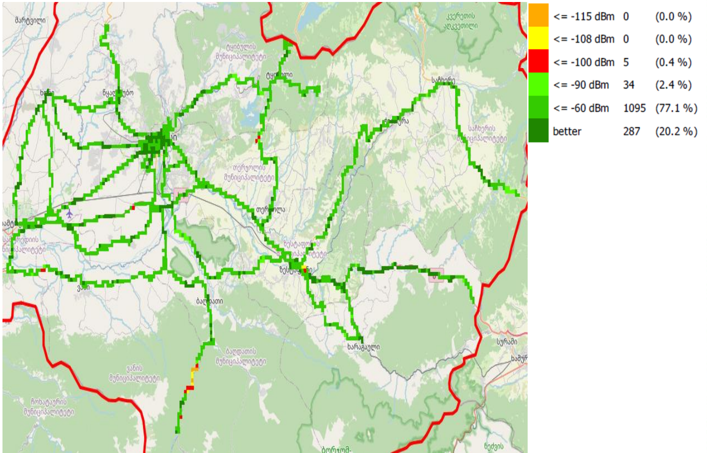
RSCP, მაგთიკომი
