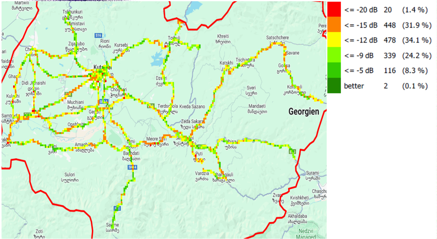
RSRQ, სოლენგეტი
