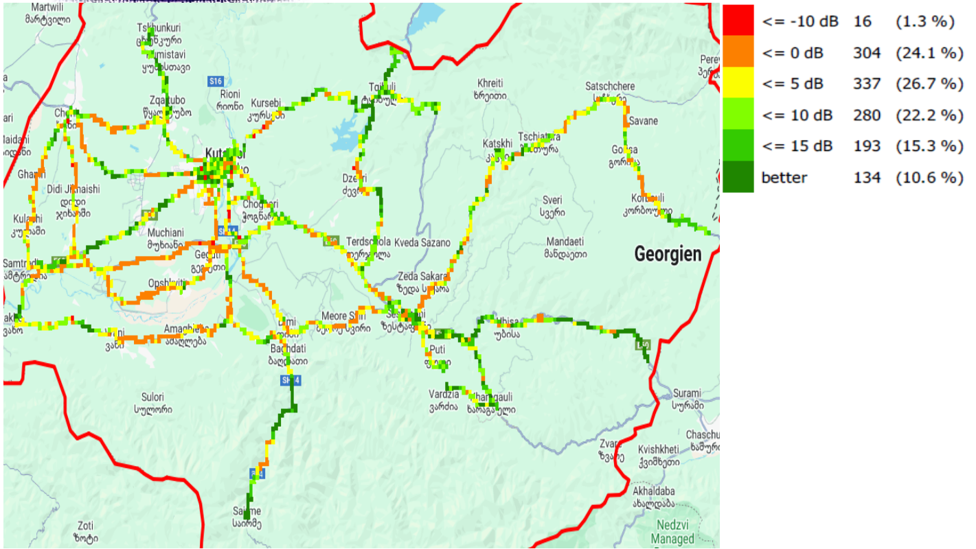
SINR, სელფი
