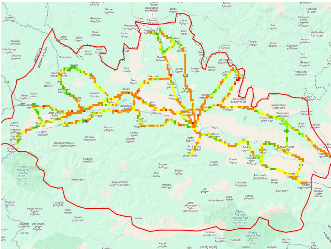
RSRQ, სელფი
