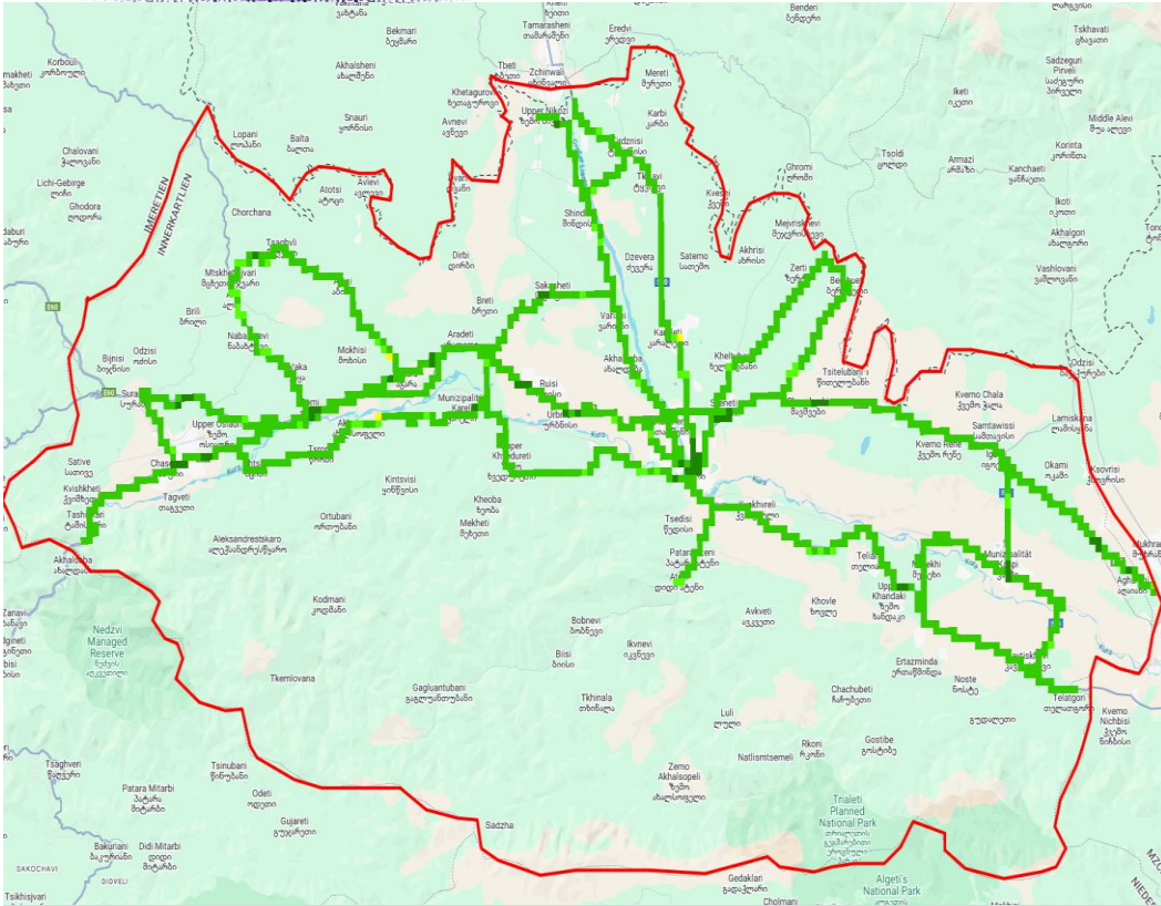
RSRP, მაგთიკომი
