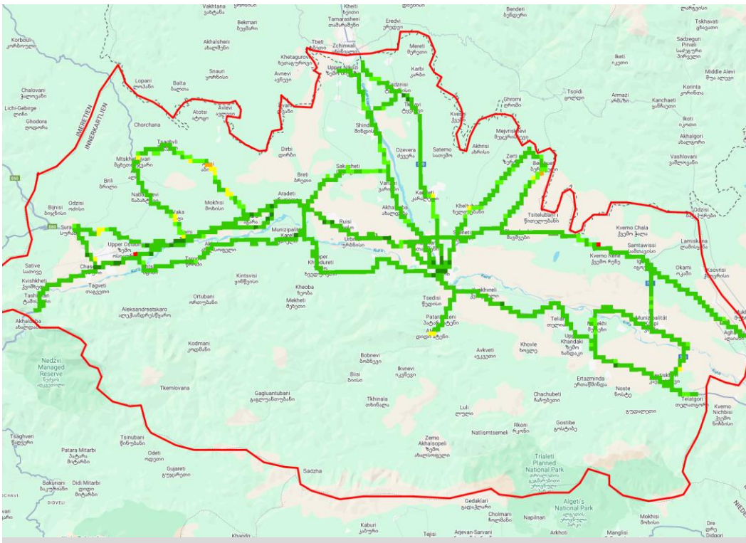
RSRP, სილქნეტი
