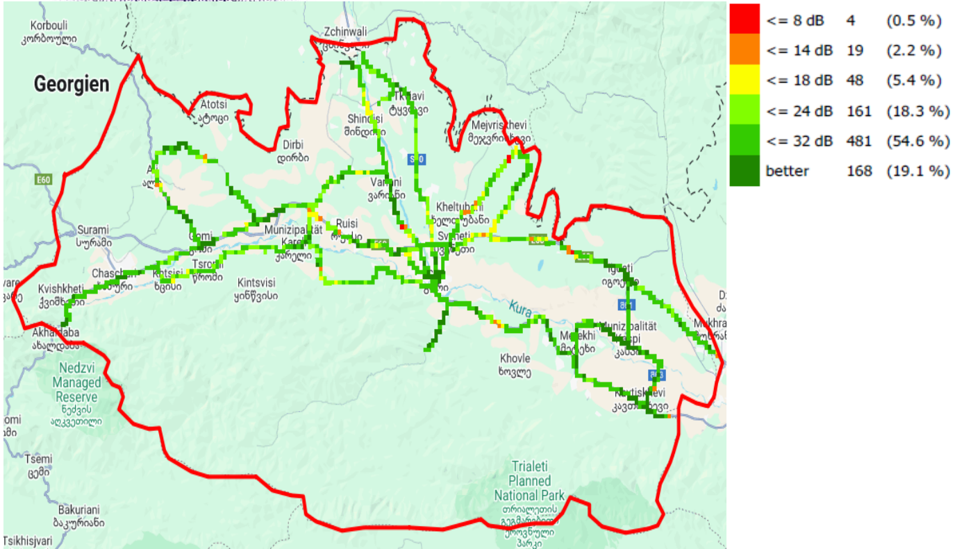
C/I, მგეტიკომი
