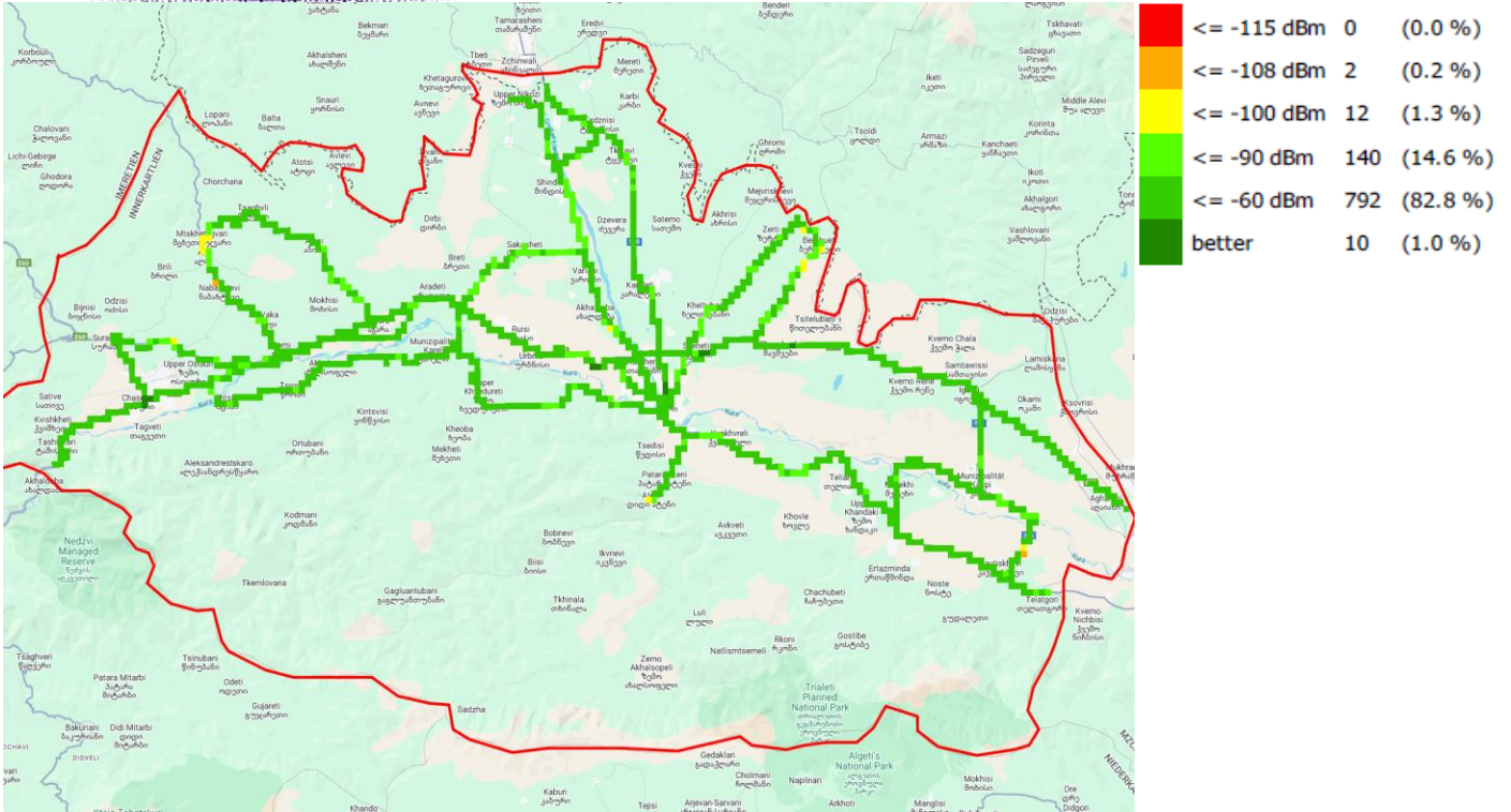
RSRP, სელვი
