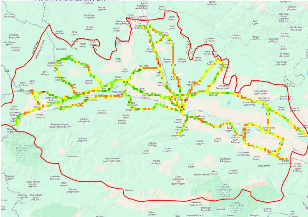
RSRQ, სოლქნეტი
