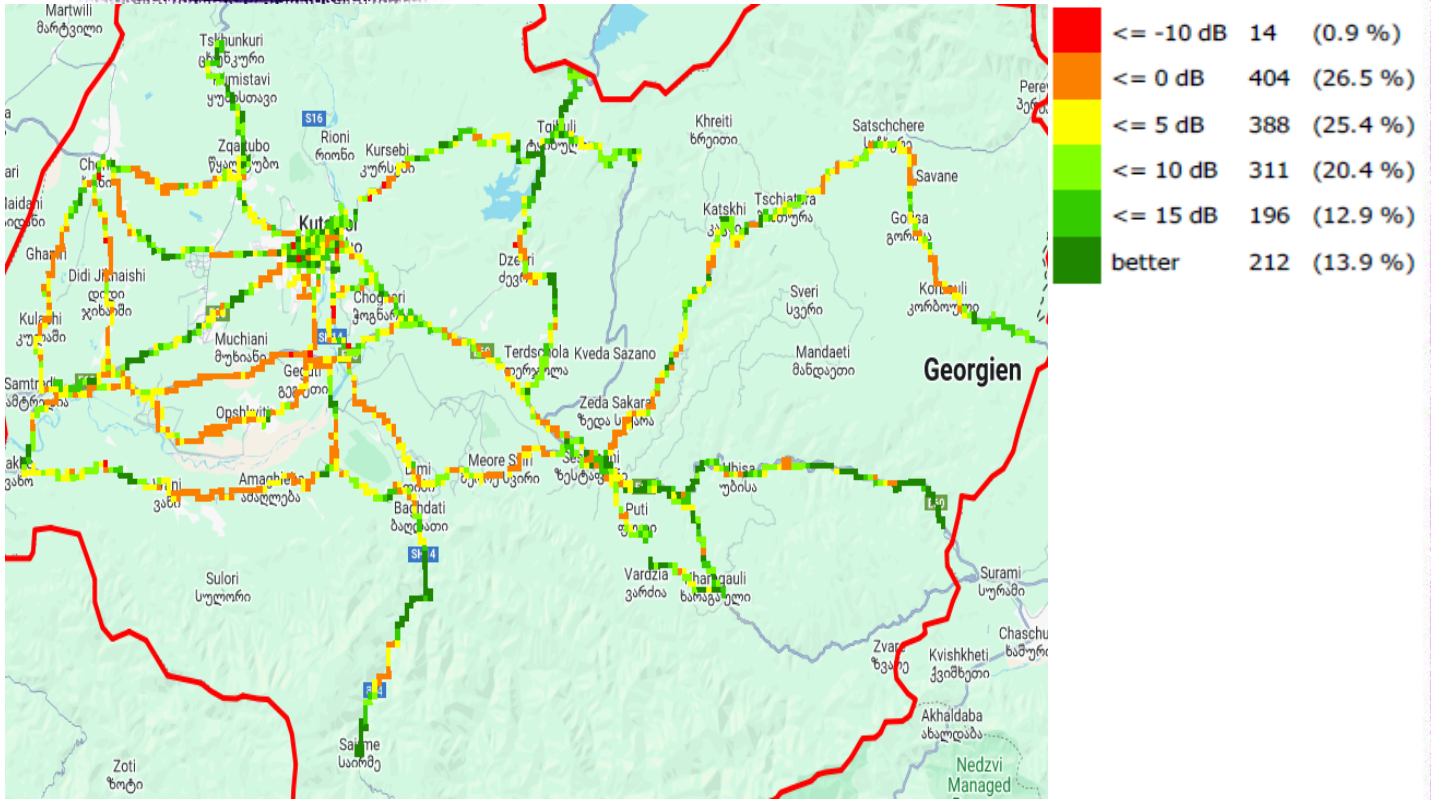
SINR, სელფი
