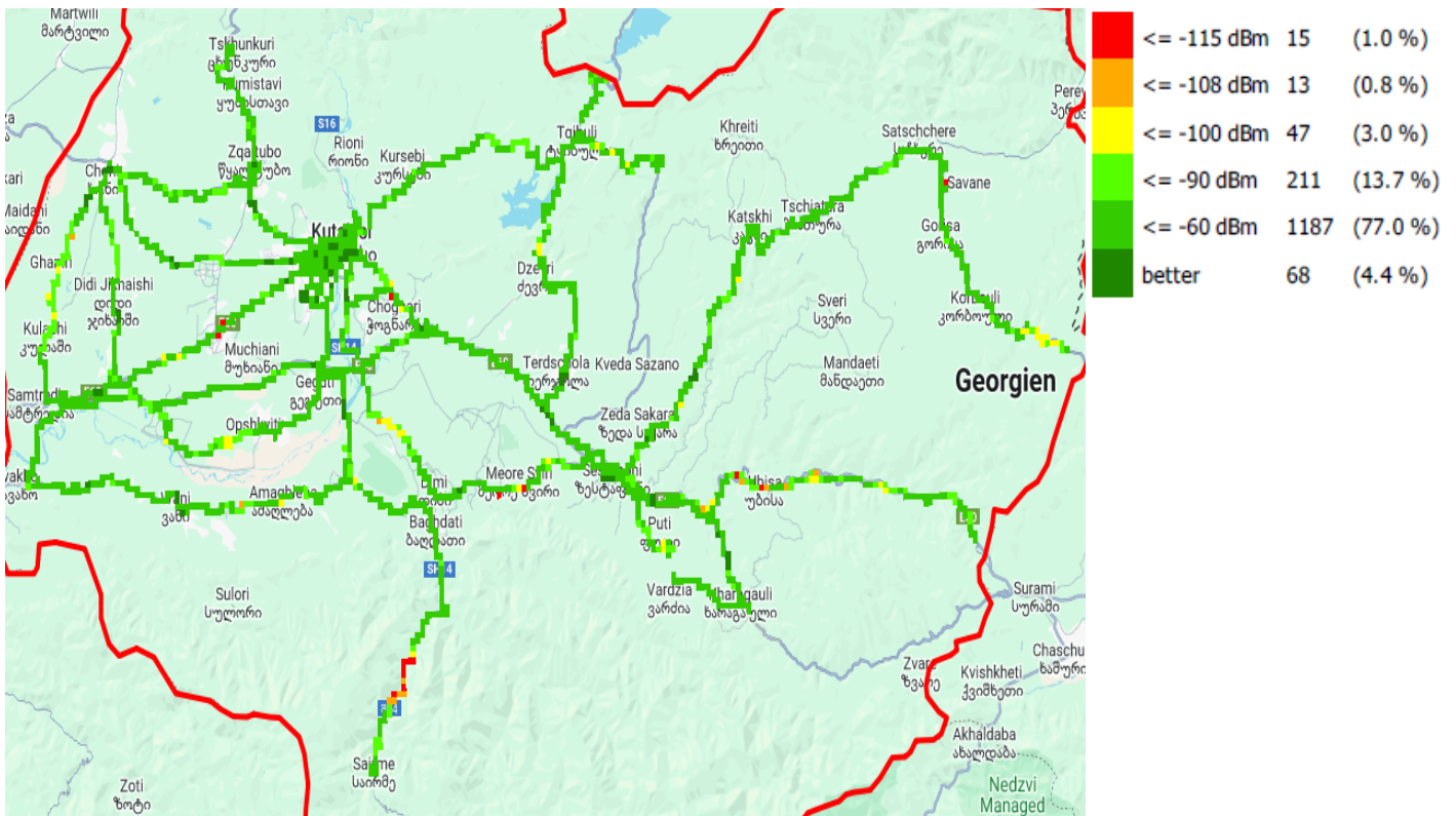
RSRP, სილქნეტი
