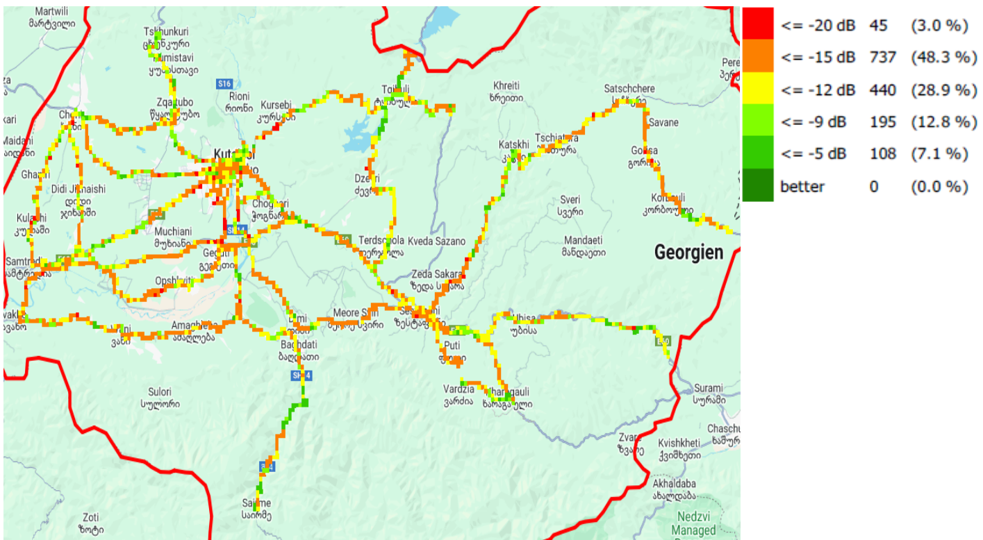
RSRQ, სელფი
