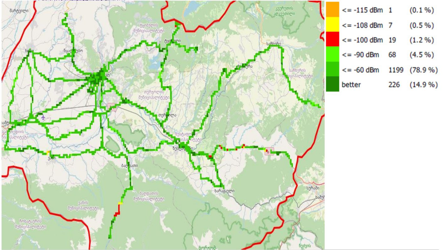
RSCP, სილქნეტი
