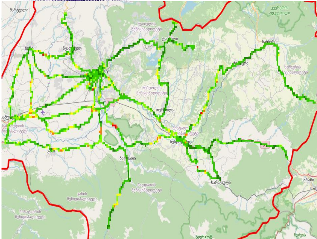
C/I, მაგთიკომი
