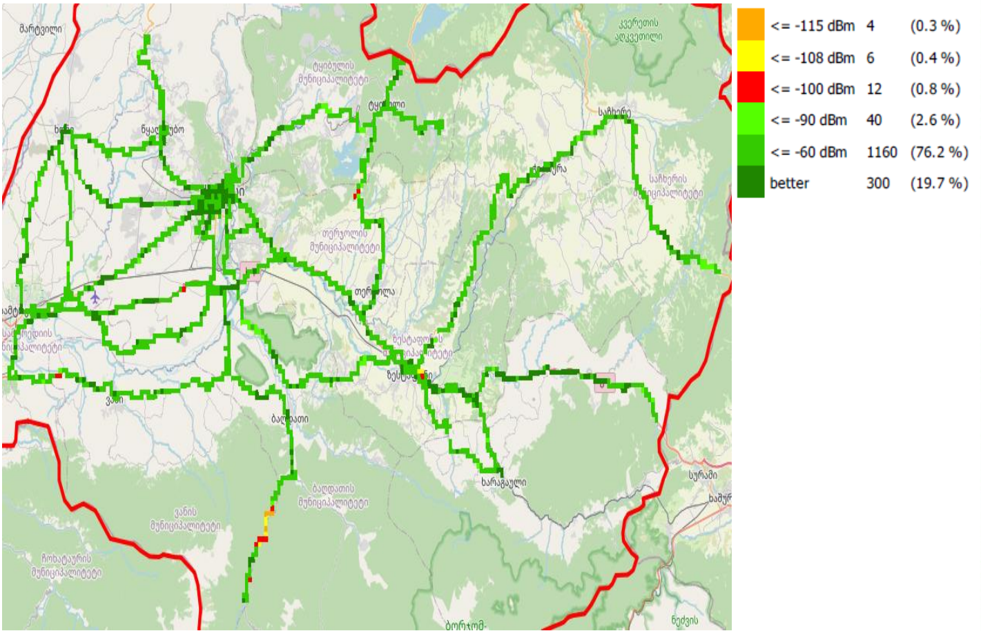
RSCP, მაგთიკომი
