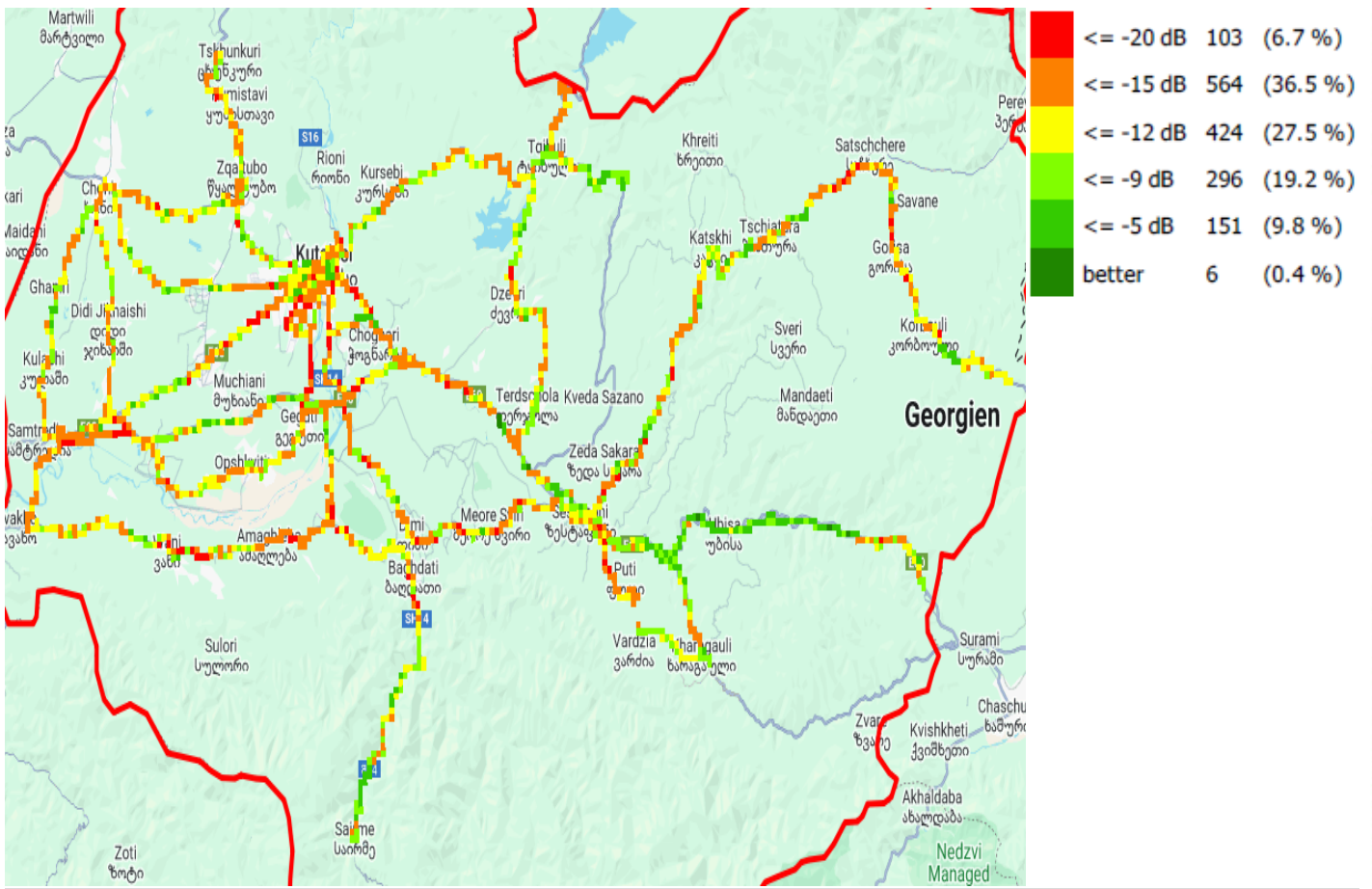
RSRQ, მაგთიკომი
