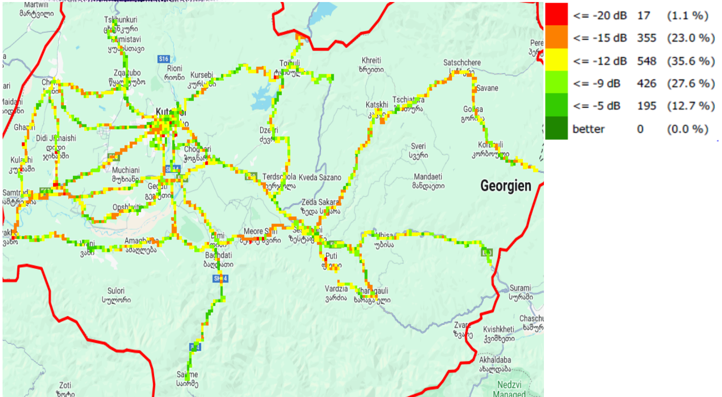
RSRQ, სილქნეტი
