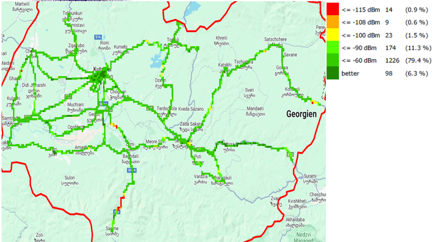
RSRP, მაგთიკომი
