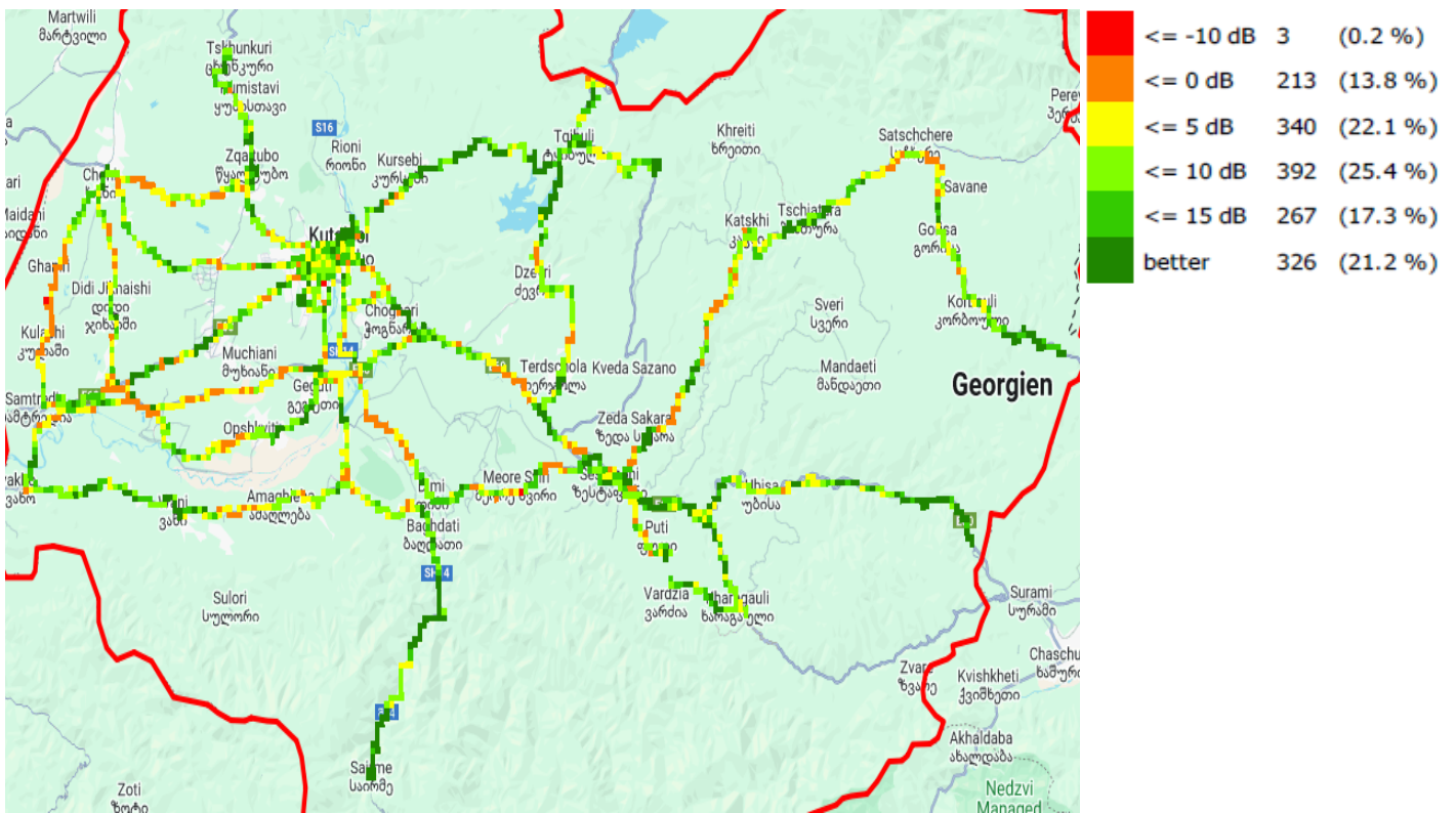
SINR, სილქნეტი
