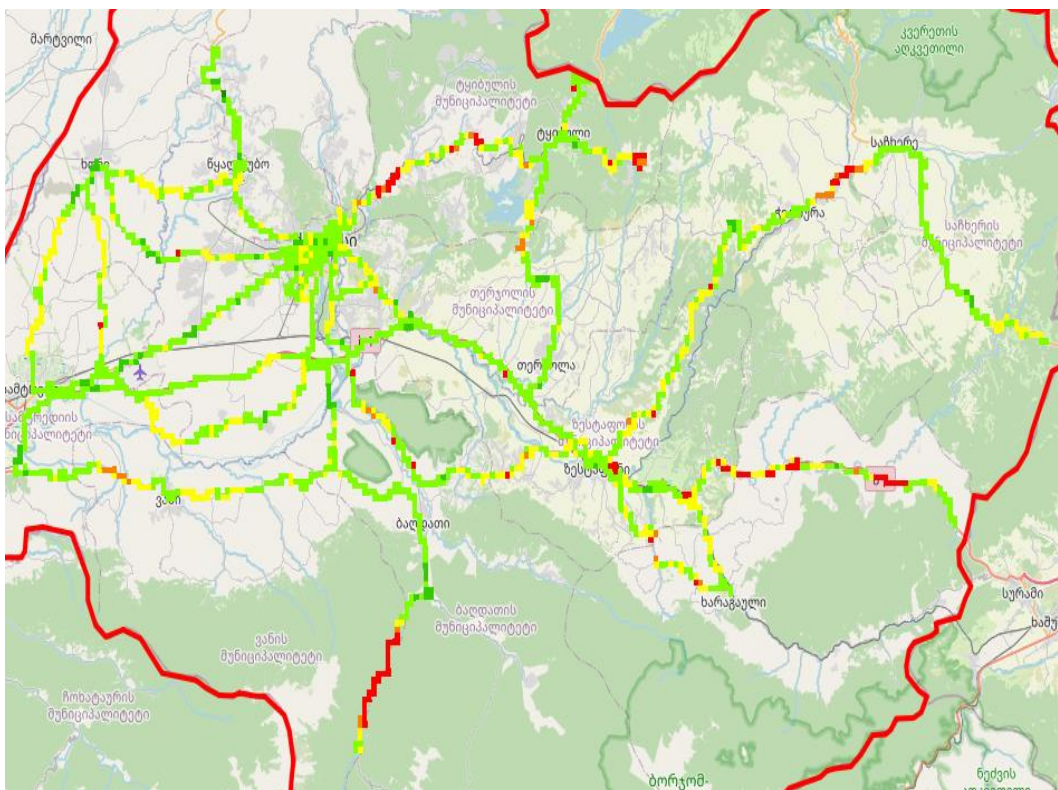
RX_LEV, სელფი
