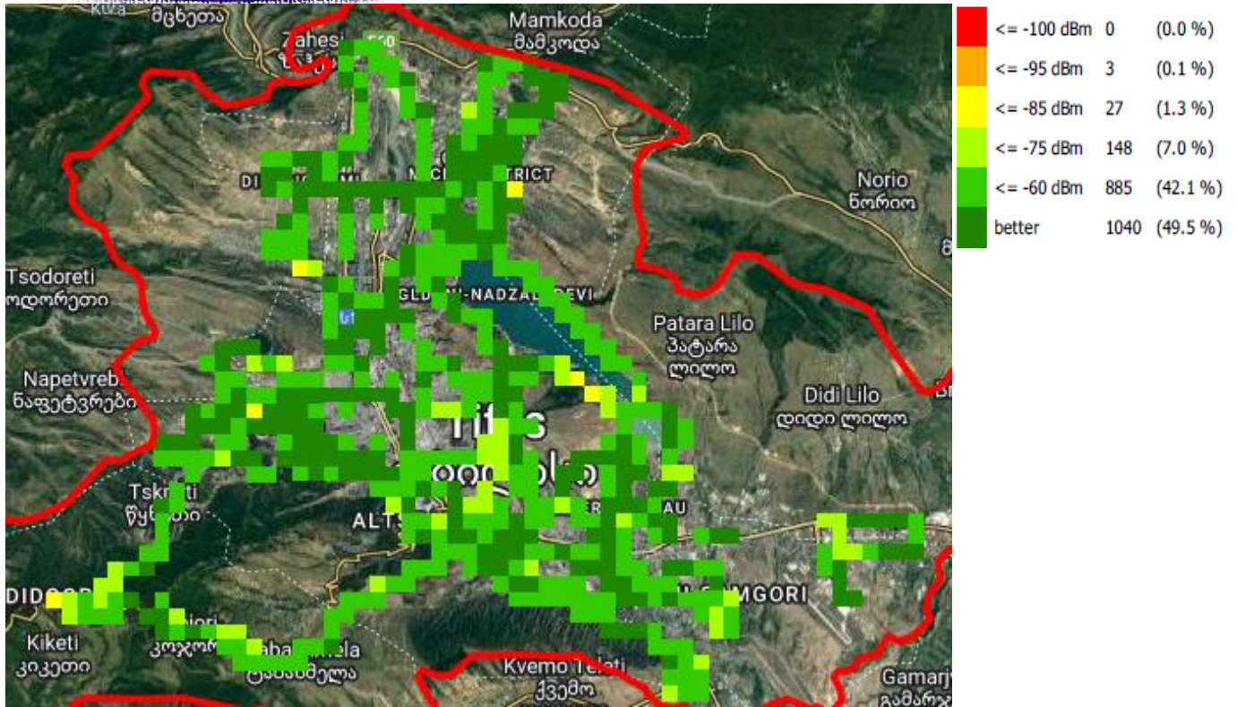
RSCP, მაგთიკომი
