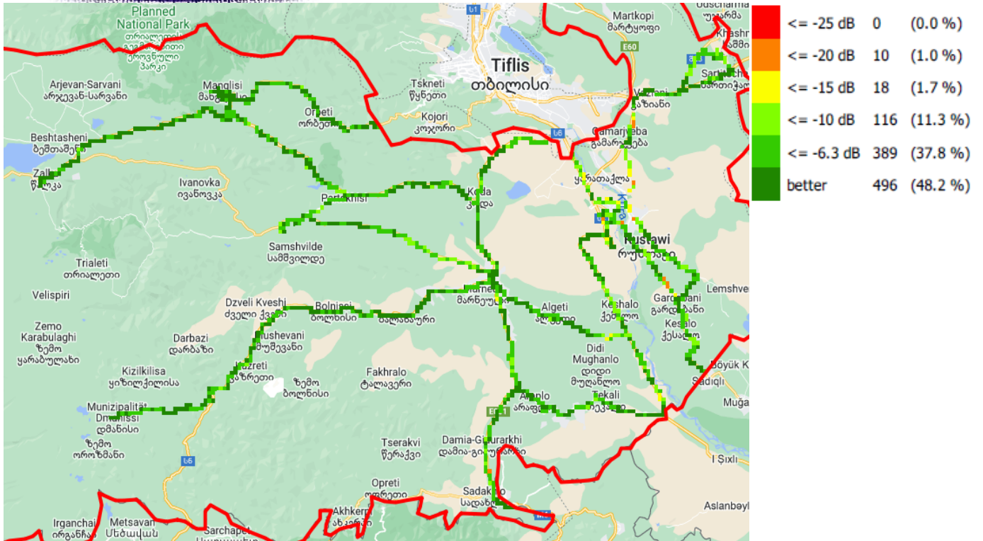
E c /I o , მატეიკომი
