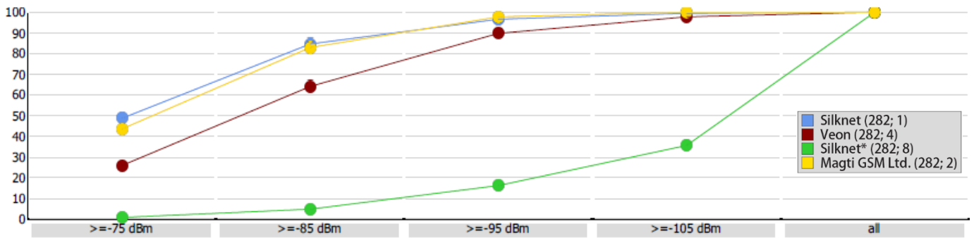
RSRP, ვიონი საქართველო
