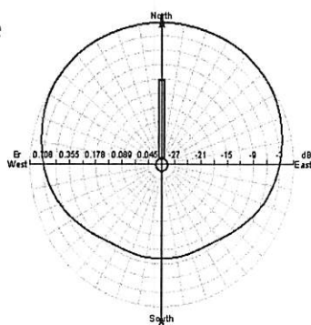
H-plane
