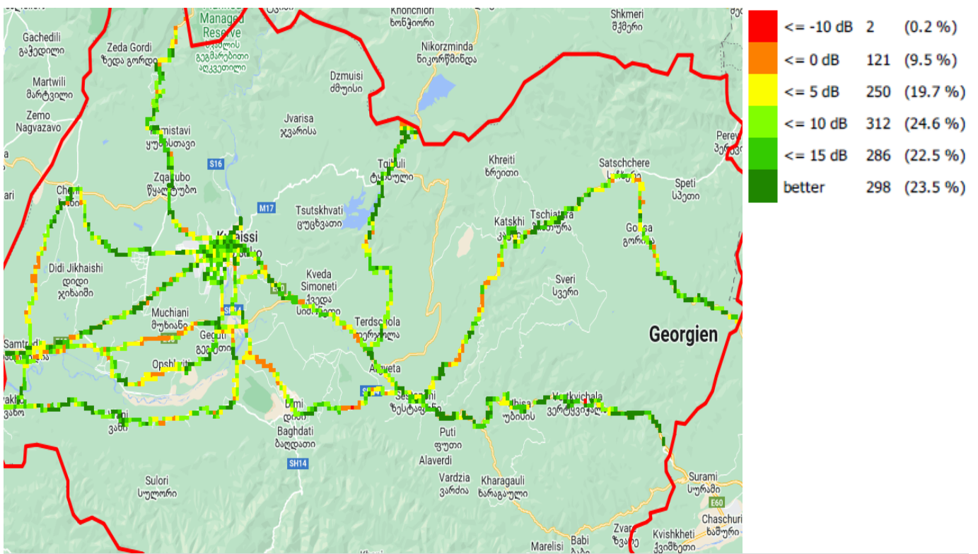
SINR, სოლქნეტი
