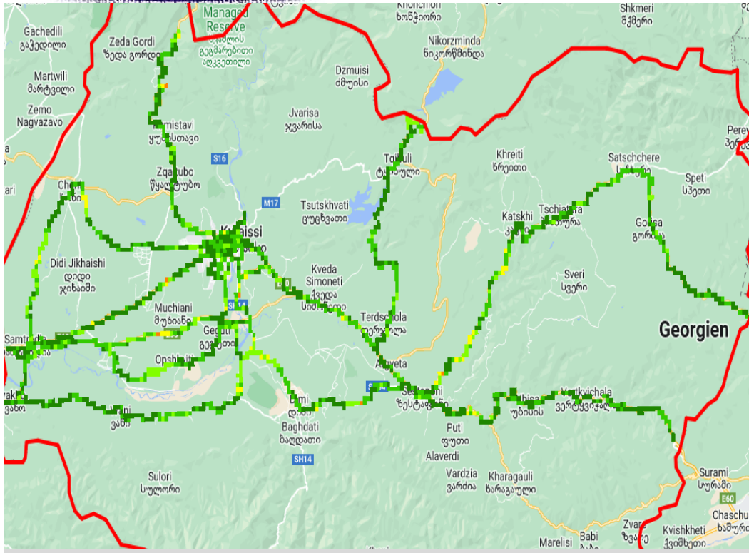
Ec/Io, სილქნეტი
