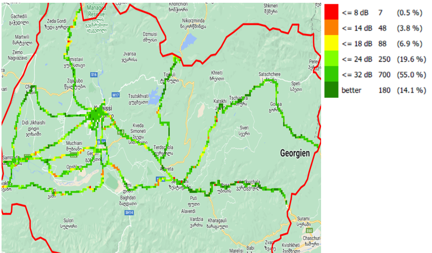
C/I, მაგთიკომი
