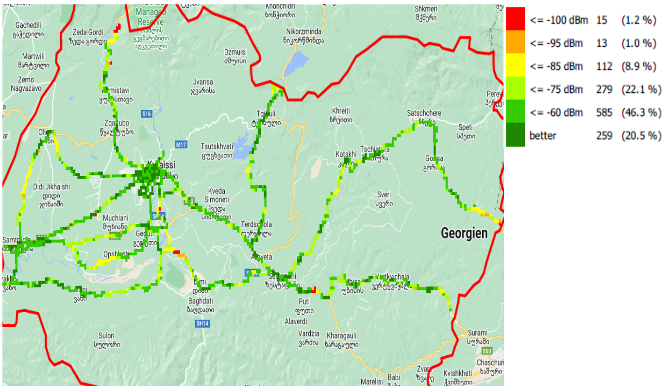
RSCP, სილქნეტი
