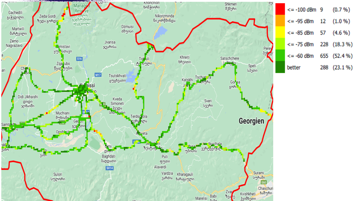
RSCP, მაგთიკომი
