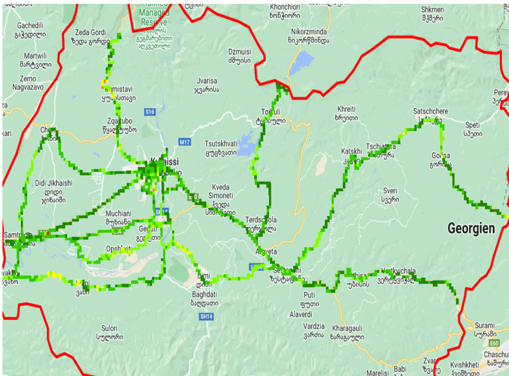
Ec/Io, ვიონი საქართველო
