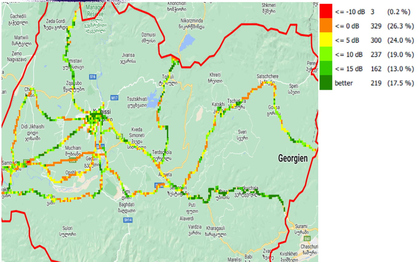
SINR, ვიონი საქართველო
