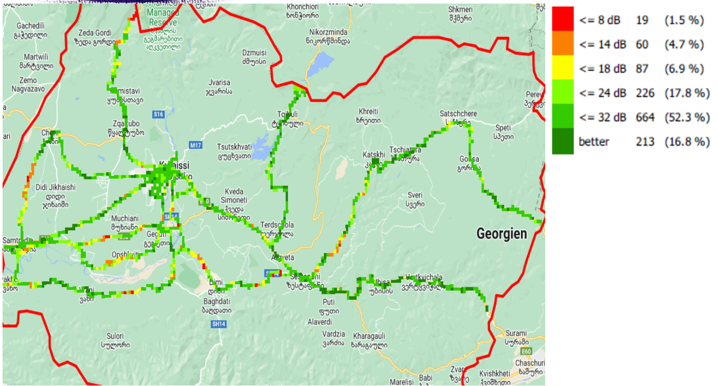
C/I, სილქნეტი
