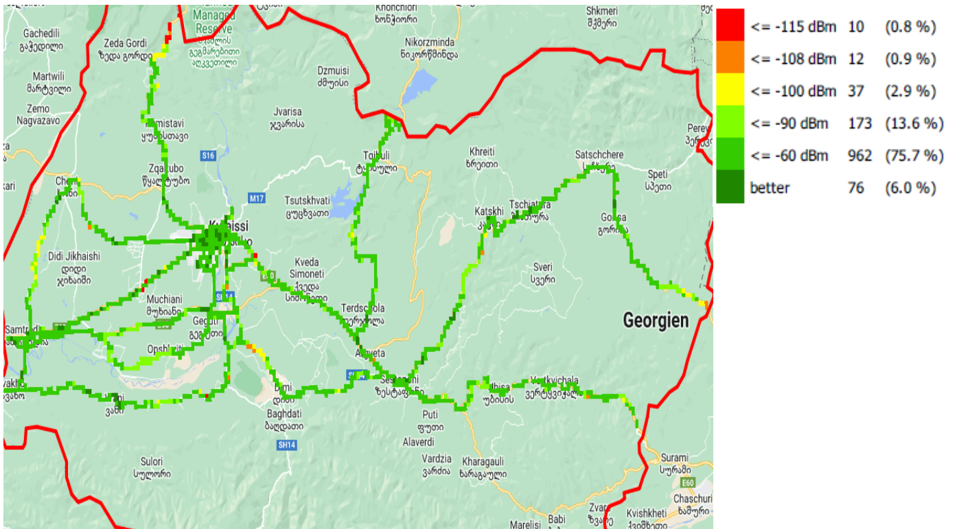
RSRP, სილქნეტი
