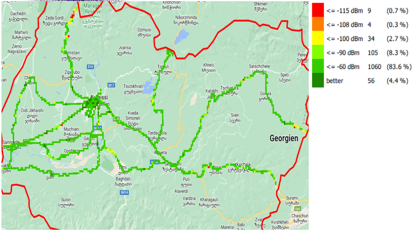
RSRP, მაგთიკომი
