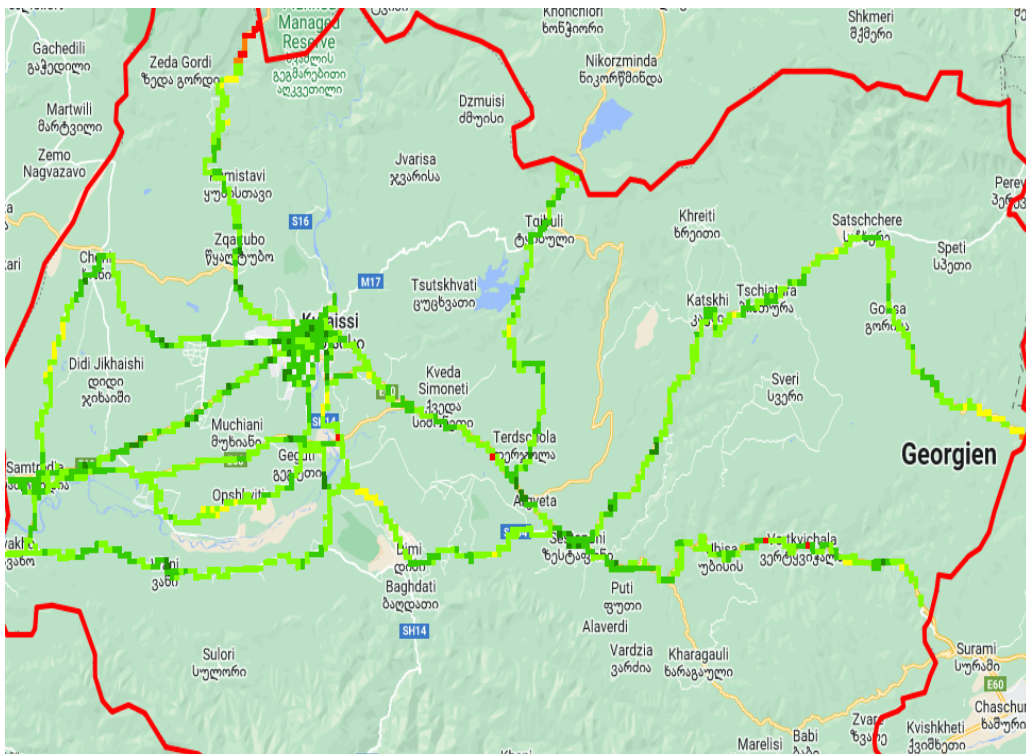
RX_LEV, სილქნეტი
