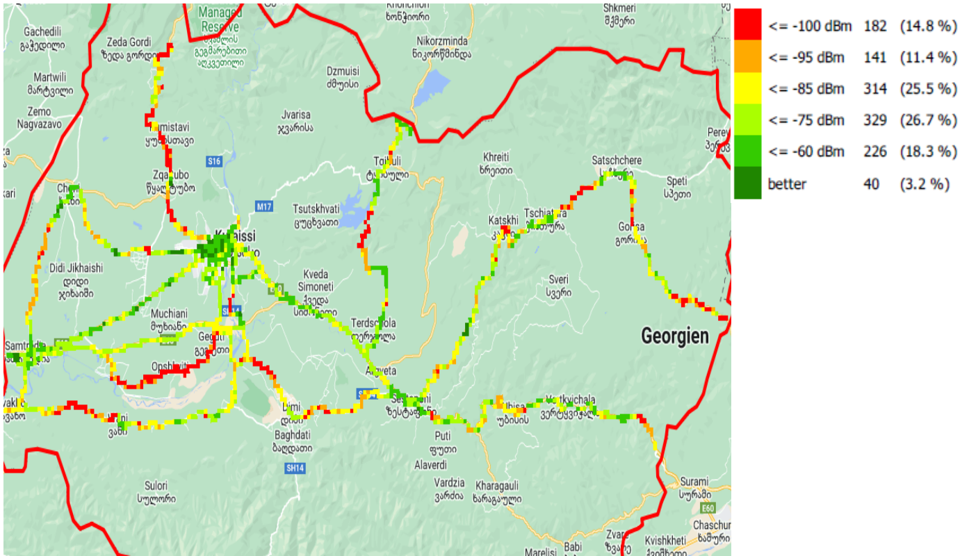
RSCP, ვიზი საქართველო
